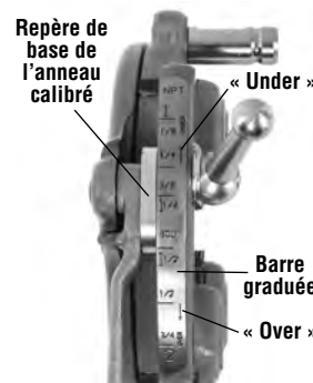
Figure 7 – Réglage du filetage
