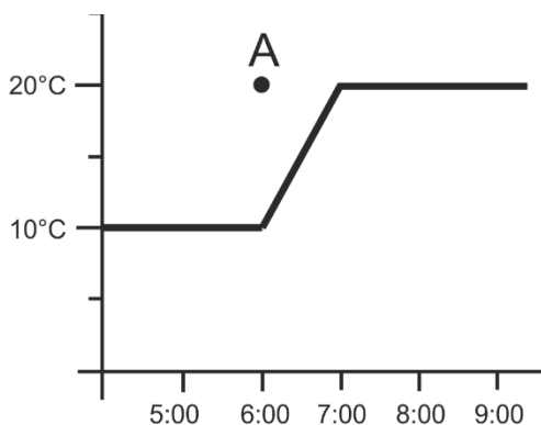
Температура помещения — выключена функция ОПТИМАЛЬНЫЙ СТАРТ:
