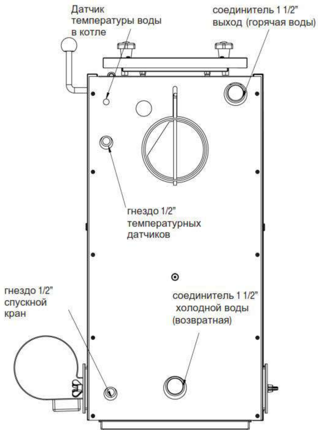
Рис. 02. Расположение и размеры отверстий котла.
