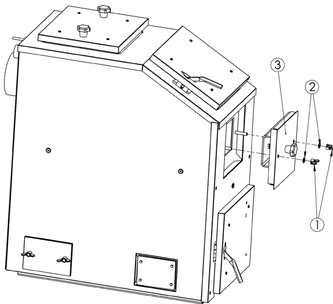
Рис. 04. Установка заглушки.
