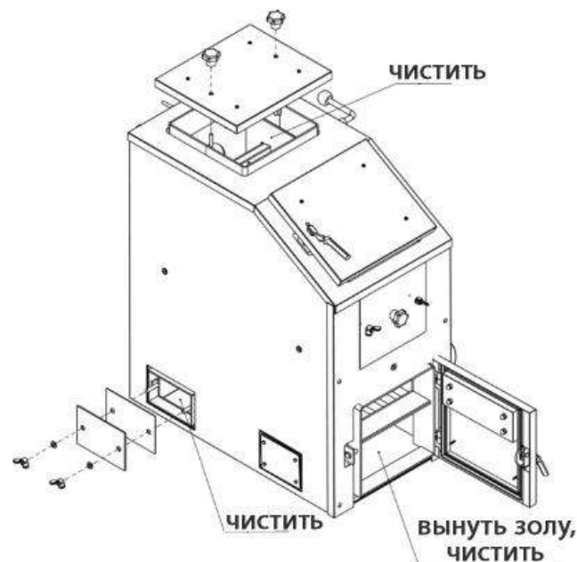
Рис. 05. Чистка котла.
