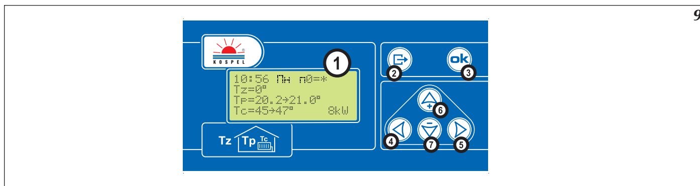
Рис.9 Панель управления EKCO.M1z
