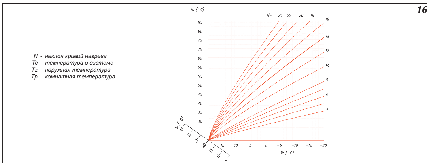
Рис. 16 Кривая нагрева
