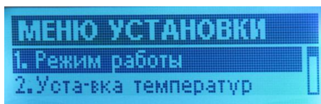
Рисунок 13 Меню установки
