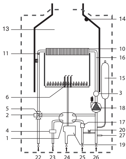
Принципиальная схема
