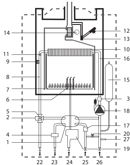
Принципиальная схема
