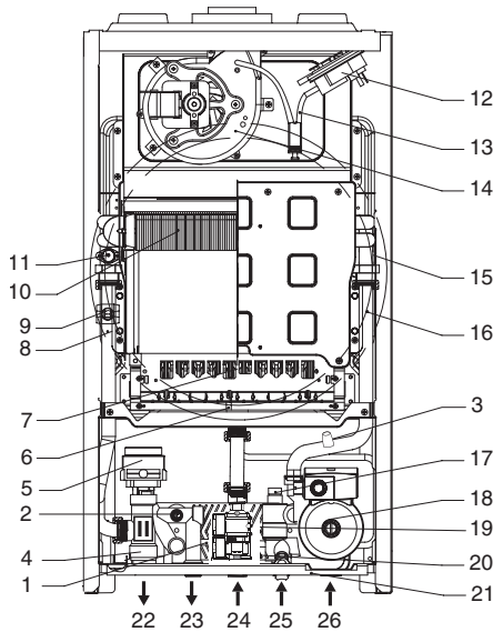
Внутренняя структура
