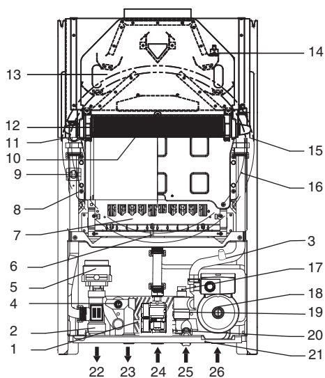
Внутренняя структура
