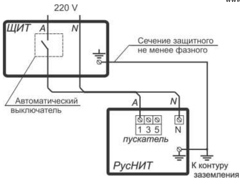
Рис.6. Схема подключения РусНИТУ205НМ,206НМ, 207НМ, 208НМ, 209НМ к однофазной сети .
