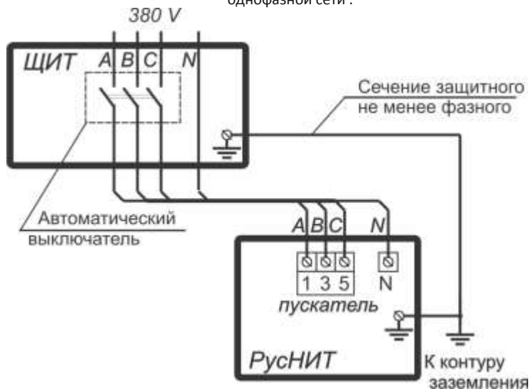
Рис.7. Схема подключения РусНИТУ206НМ, 207НМ, 208НМ, 209НМ к трёхфазной сети.
