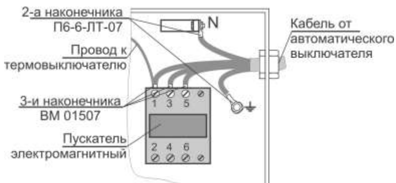
Рис.4. Подключение РусНИТУ205НМ, 206НМ, 207НМ, 208НМ, 209НМ к однофазной сети.
