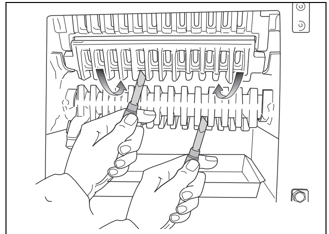
Рис. 21 Чистка откидной решётку инструментом
