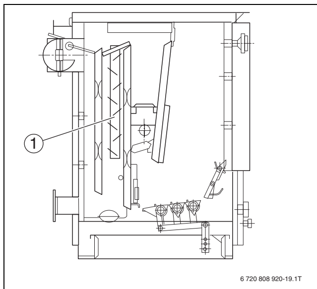
Рис. 16 Турбулятор в тракте дымовых газов
