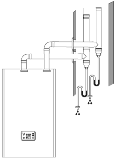
Минимальные внутренние размеры камеры для прохода двух дымоходов, диаметр 50 мм
