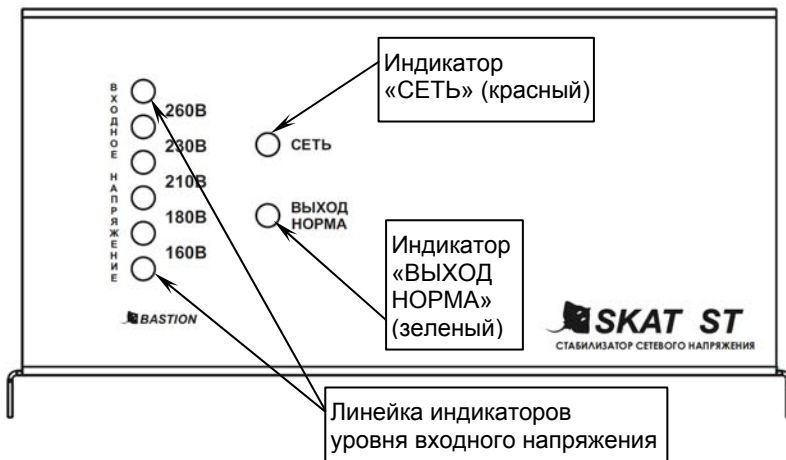
Рисунок 2 – Вид стабилизатора со стороны индикации
