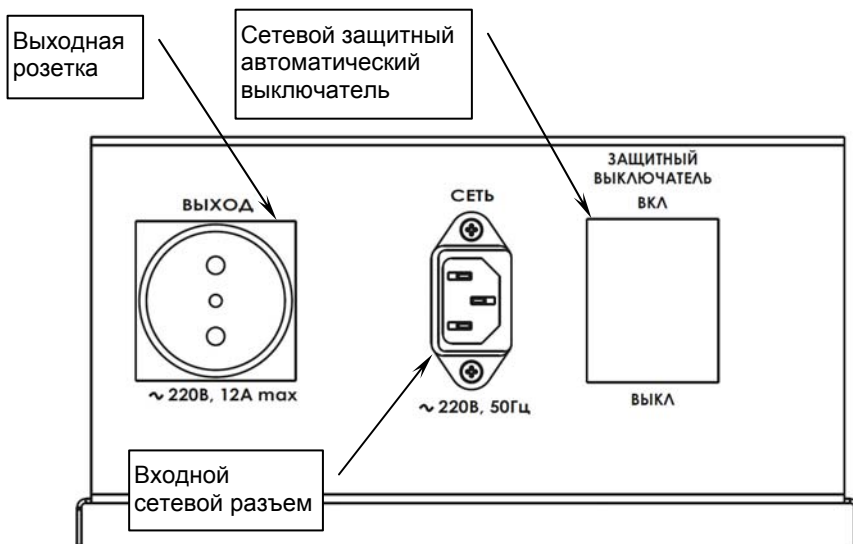
Рисунок 3 – Вид стабилизатора со стороны подключения
