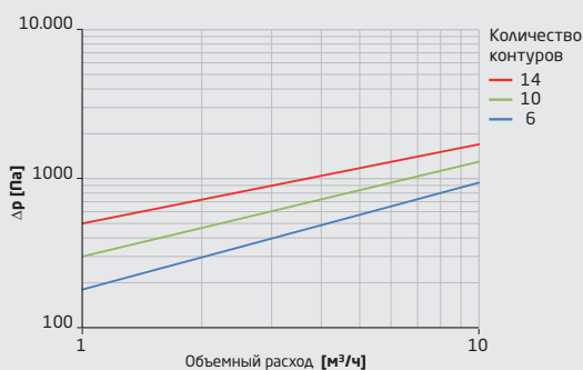
Рис. 2. Диаграмма потерь давления, тип 120/80
