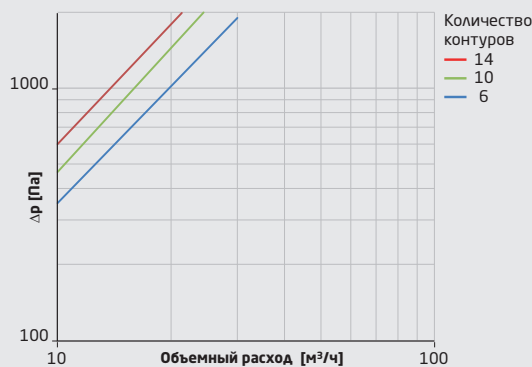
Рис. 5. Диаграмма потерь давления, тип 200/120
