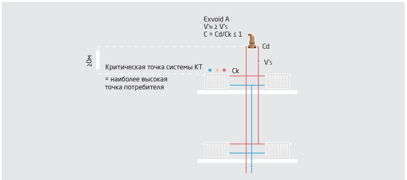
Рис. 144: Сепаратор микропузырьков Exvoid A устанавливается в наиболее высокую точку
