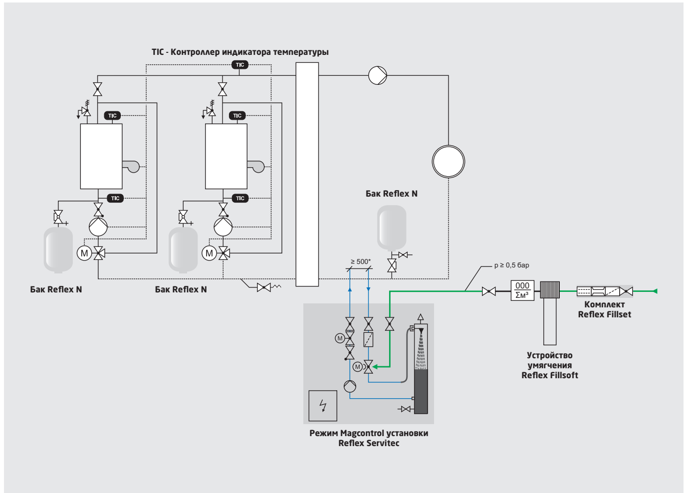
Рис. 93. Режим Magcontrol в установке с несколькими котлами, гидравлической стрелкой и МБР
