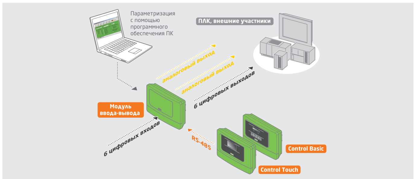
Рис. 135: Модуль ввода-вывода - соединение с ПЛК и внешними участниками с помощью цифровых и аналоговых устройств сопряжения
