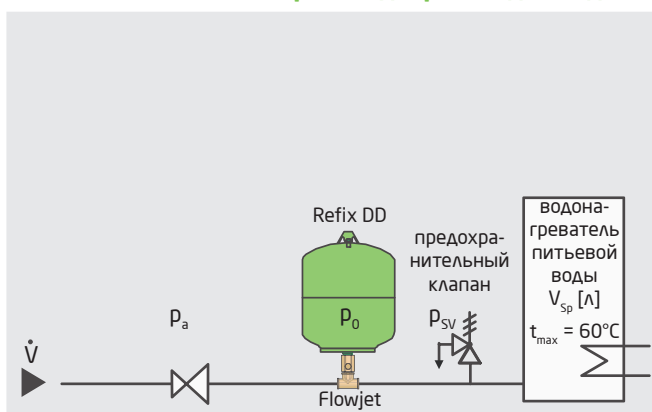
Рис. 58. Быстрый выбор баков для водонагревателя
