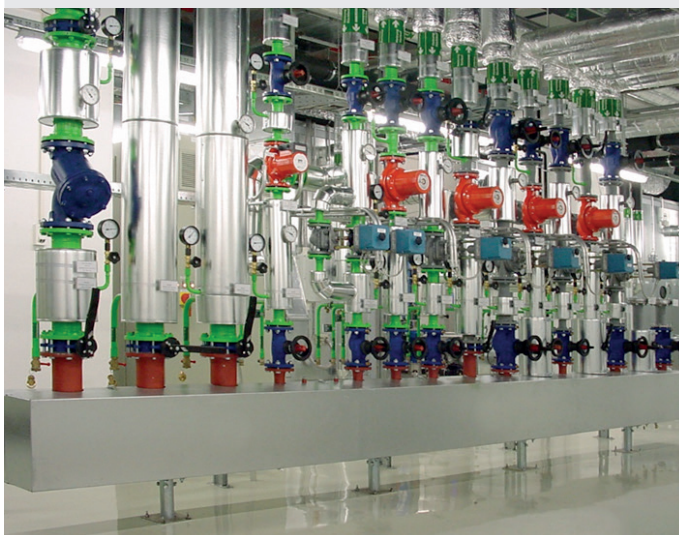
Рис. 16. Компактный монтаж с синусоидальным компактным коллектором
