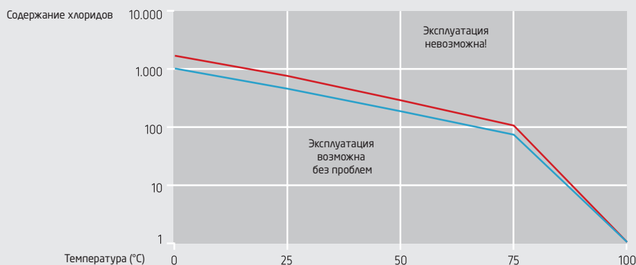
Рис. 45. Предельные значения содержания хлоридов при эксплуатации медно-паянных пластинчатых теплообменников
