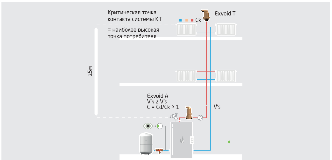
Рис. 145: Сепаратор микропузырьков Exvoid A устанавливается ниже наиболее высокой точки
