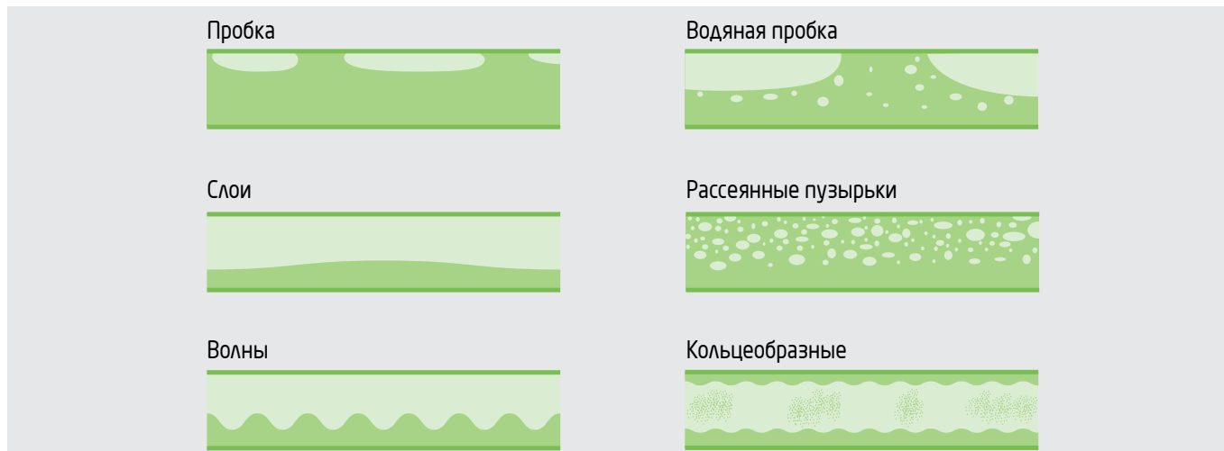
Рис. 83. Характер воздушных включений в горизонтальных трубопроводах [Ghajar, 2005]
