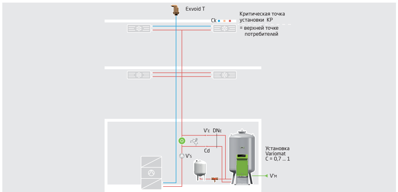
Рис. 96. Станция поддержания давления Reflex Variomat с атмосферной дегазацией в системе холодоснабжения
