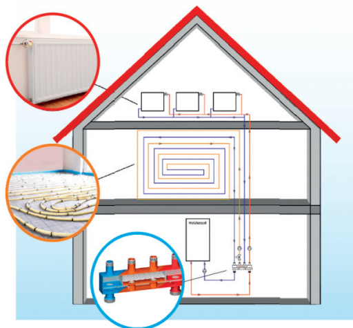
Рис. 41. Sinus MultiFlow Domestic в системе отопления одноквартирного дома
