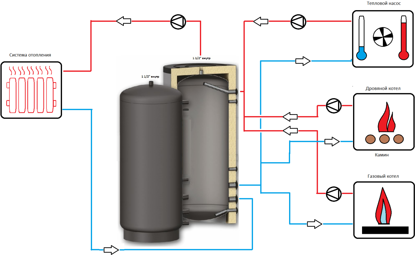
Принципиальная схема работы бака серии ET
