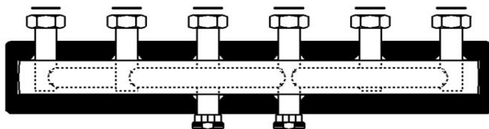
Рис.5 Коллектор до 3 отопительных контуров, нержавеющая сталь Арт 66301.41D
