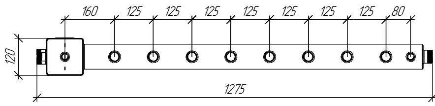
Монтажные размеры
