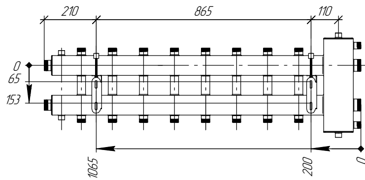
Монтажные размеры
