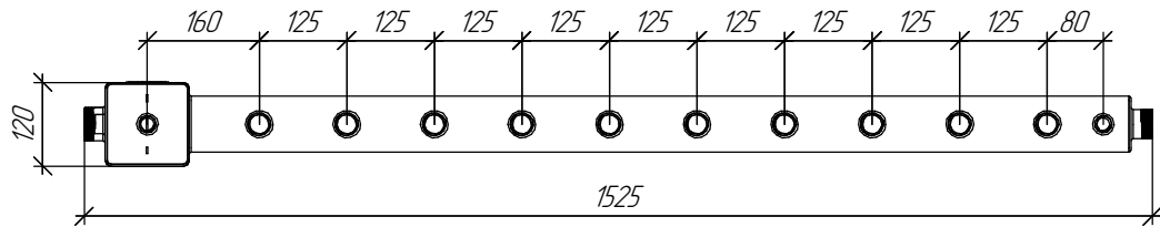
Монтажные размеры
