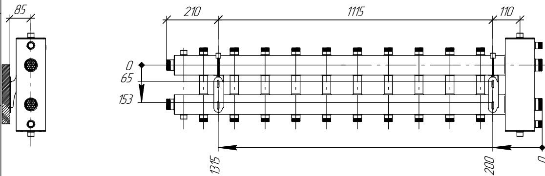
Монтажные размеры
