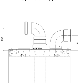
Раздельный воздухопровод и дымоотвод
