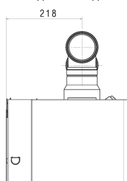
Раздельный воздухопровод и дымоотвод
