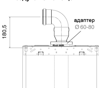
Дымоход при заборе воздуха из помещения
