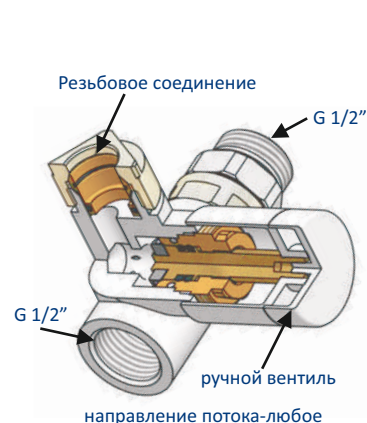
Клапан с ручным вентилем
