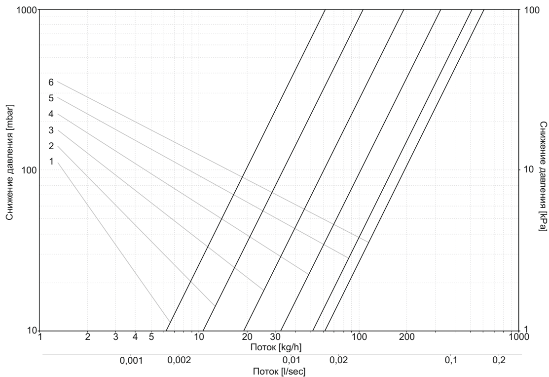
Диаграмма потока теплоносителя для вкладок 603000006, 603000007
