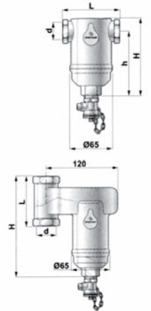
Вертикальное подсоединение
