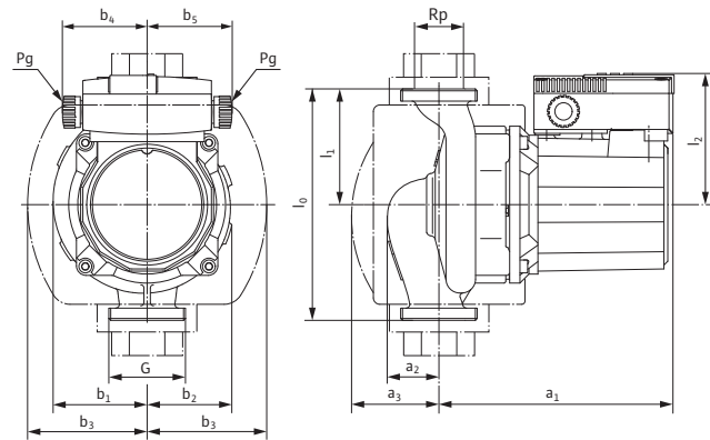
Габаритный чертежВ
