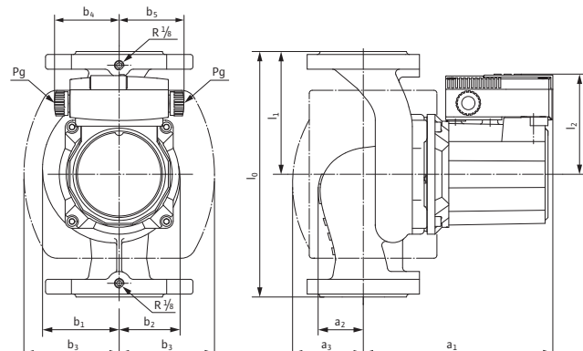
Габаритный чертежD
