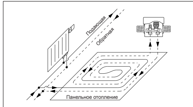
Схема монтажа для регулирования темп. панельного отопления посредством ограничения темп. обратного потока
