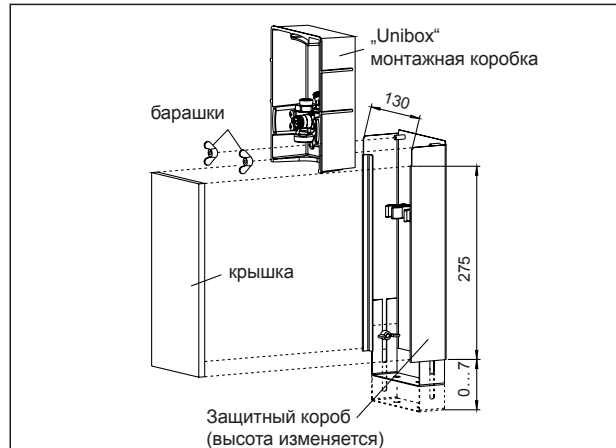
Размеры защитного короба арт. № 102 26 52
