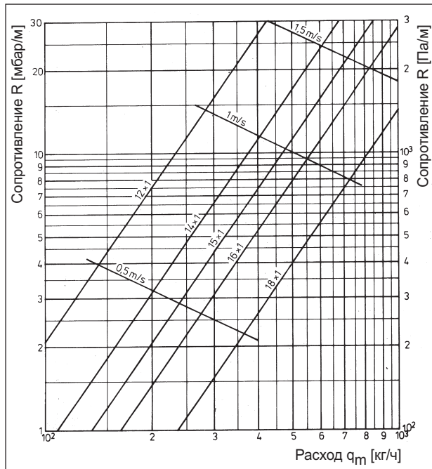
Диаграмма 15 Мягкая стальная труба Сопrotивление R в мбар/м
