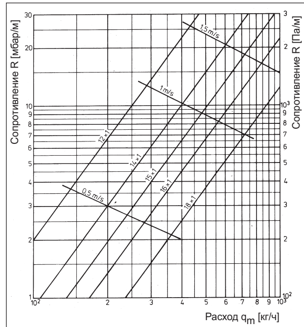
Диаграмма 16 Медная труба Сопrotивление R в мбар/м
