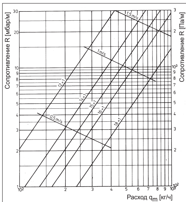
Диаграмма 15 Мягкая стальная труба Сопротивление R в мбар/м
