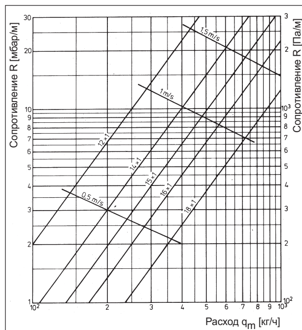
Диаграмма 16 Медная труба Сопротивление R в мбар/м
