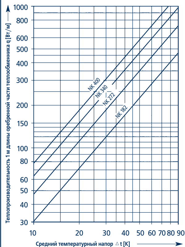
Теплопроизводительность прибора высотой 120 мм
