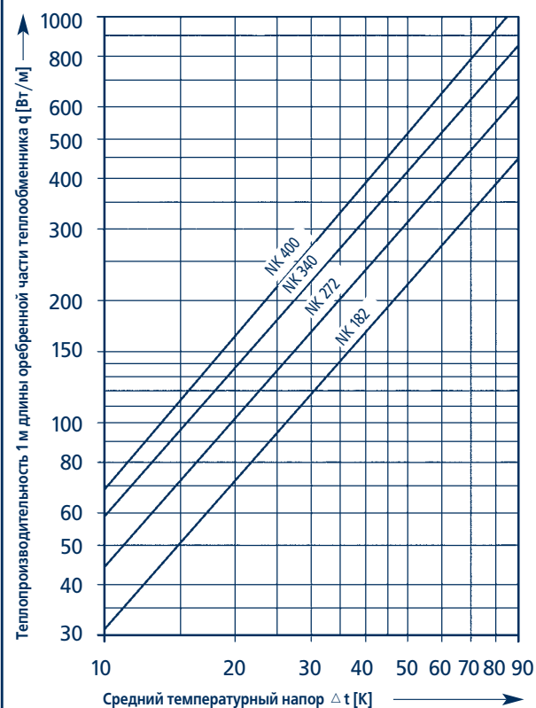
Теплопроизводительность прибора высотой 92 мм
