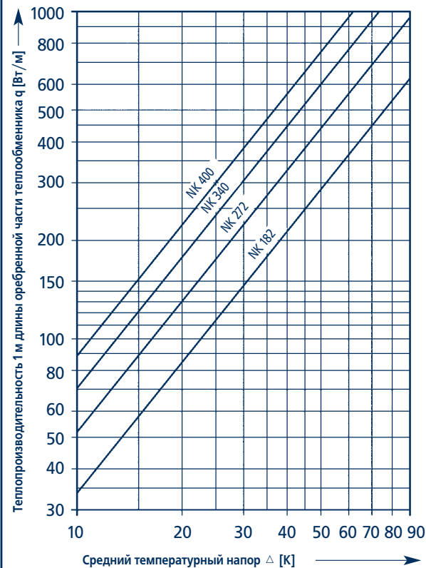
Теплопроизводительность прибора высотой 200 мм
