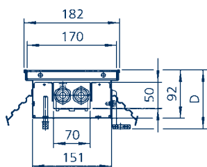
Вид в разрезе. Канал высотой 92 мм, пример монтажа с рулонной решеткой.
