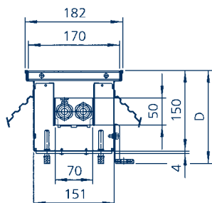
Вид в разрезе. Канал высотой 150 мм с ножками, устойчивыми к нагрузкам, возникающим при движении (ходьбе) по прибору (дополнительная принадлежность), пример монтажа с рулонной решеткой.
