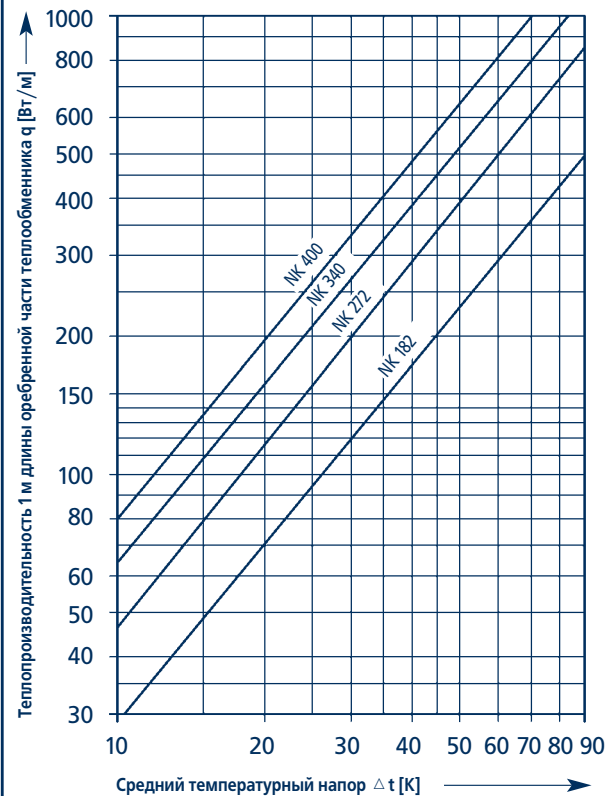
Теплопроизводительность прибора высотой 150 мм
