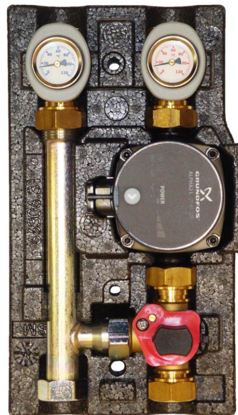
Насосно-смесительный модуль ECO МК DN20
