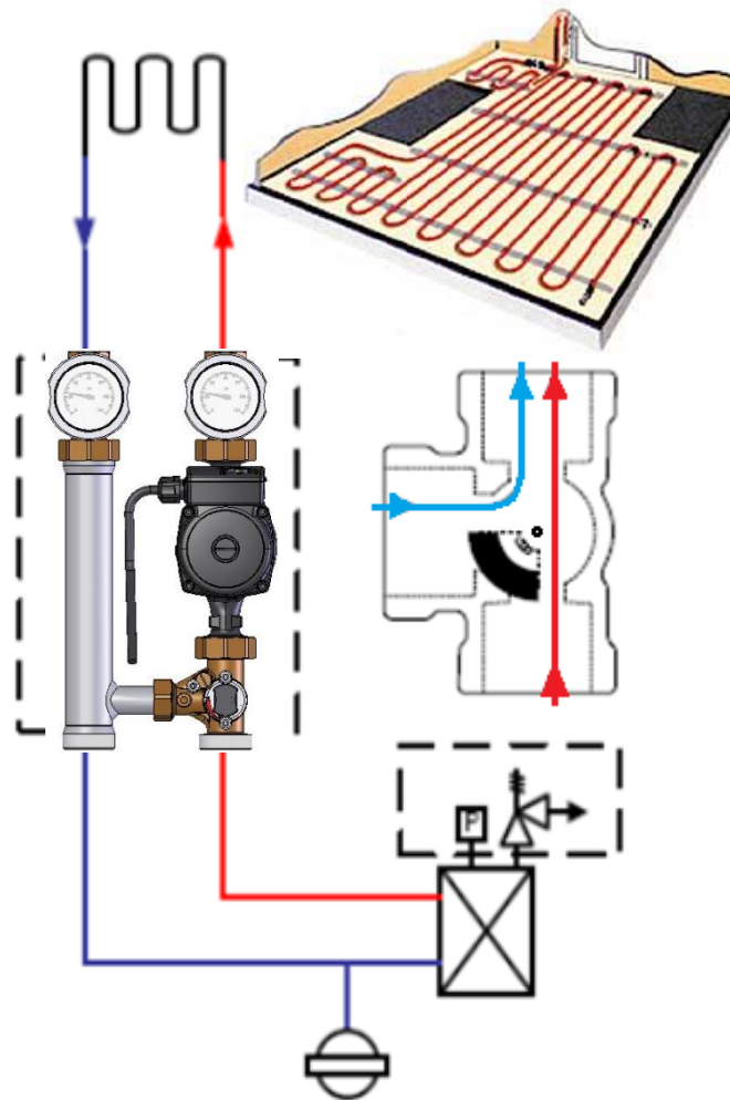
Насосно-смесительный модуль ECO MK DN20
