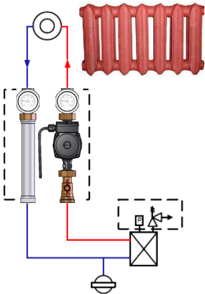
Насосный модуль ECO DK DN20
