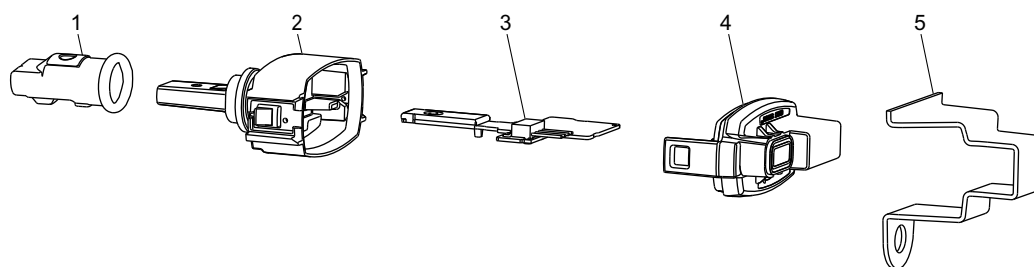
Рис. 48 Датчик
