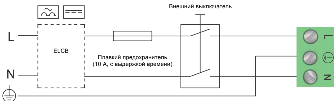
Рис. 52 Пример типового подключения, 1 x 230 В ± 10 %, 50/60 Гц
