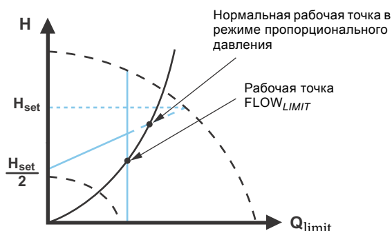
Рис. 28 Регулирование по пропорциональному давлению с функцией FLOW LIMIT
