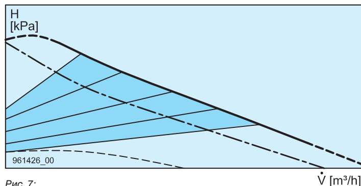
Рис. 7: Ограничение мощности для насосов с электрическим управлением
