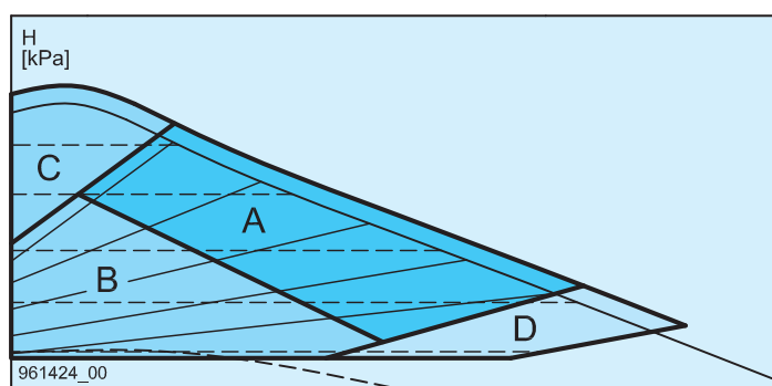
Рис.: Выбор регулируемых насосов
