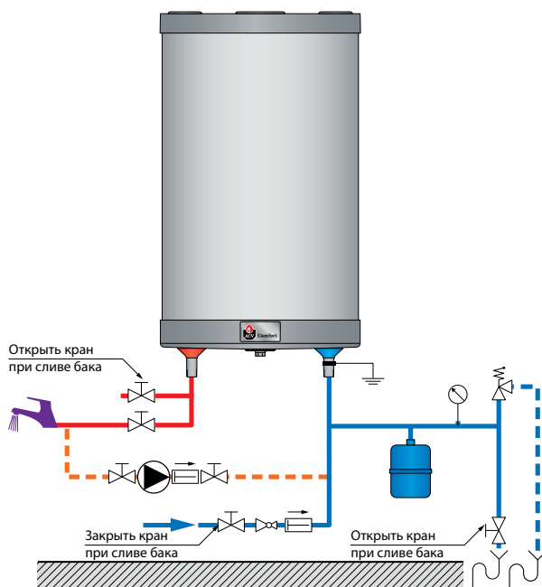
Настенный монтаж
