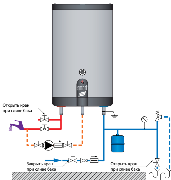
Настенный монтаж
