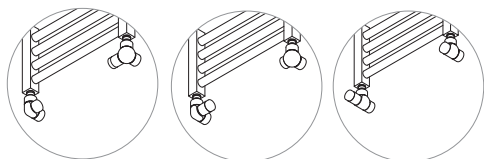
Комплект LUX с ручной регулировкой осевой правый
