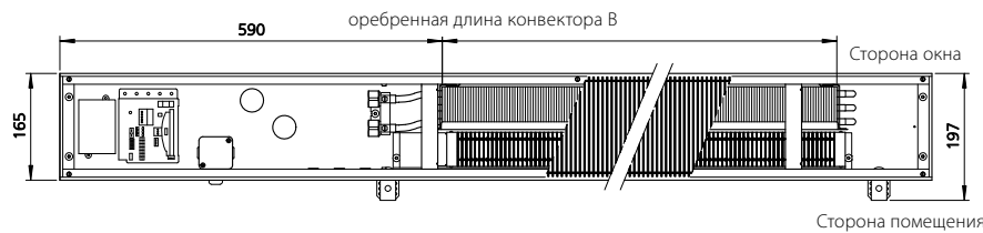
Вид сверху (вид без защитной крышки)
