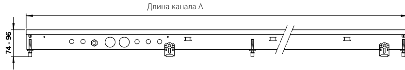
Вид спереди
