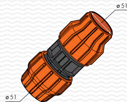
Муфта соед. для шланга PP 51 x 51 (арт. 9259)
