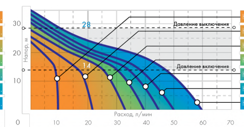
«ДЖАМБО» 60/35 П (Ч, Н)
