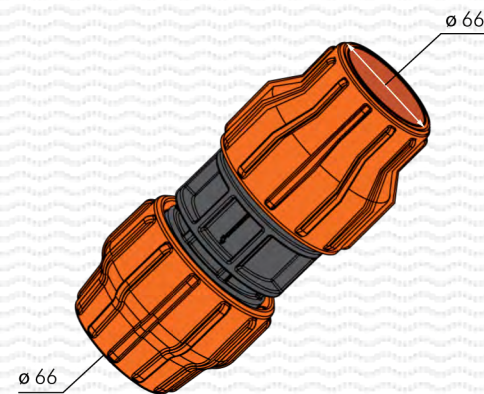
Муфта соед. для шланга PP 66 x 66 (арт. 9260)
