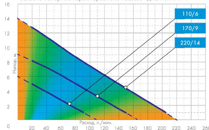
Расходно-напорные характеристики насосов «ДРЕНАЖНИК»:
