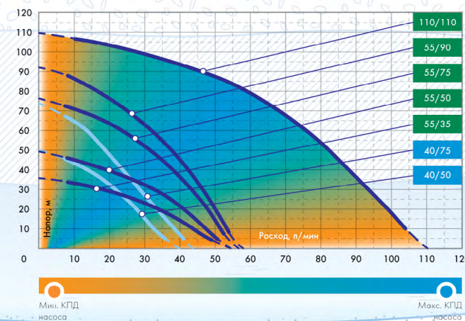
Расходно-напорные характеристики насосов «ВОДОМЕТ»:
