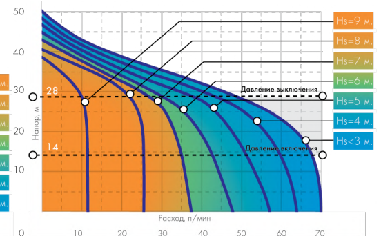
«ДЖАМБО» 70/50 П (Ч, Н)
