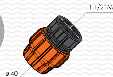
Муфта комб. для шланга PP 40 x 1 1/2" М (арт. 9248)
