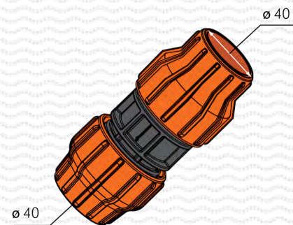
Муфта соед. для шланга PP 40 x 40 (арт. 9258)
