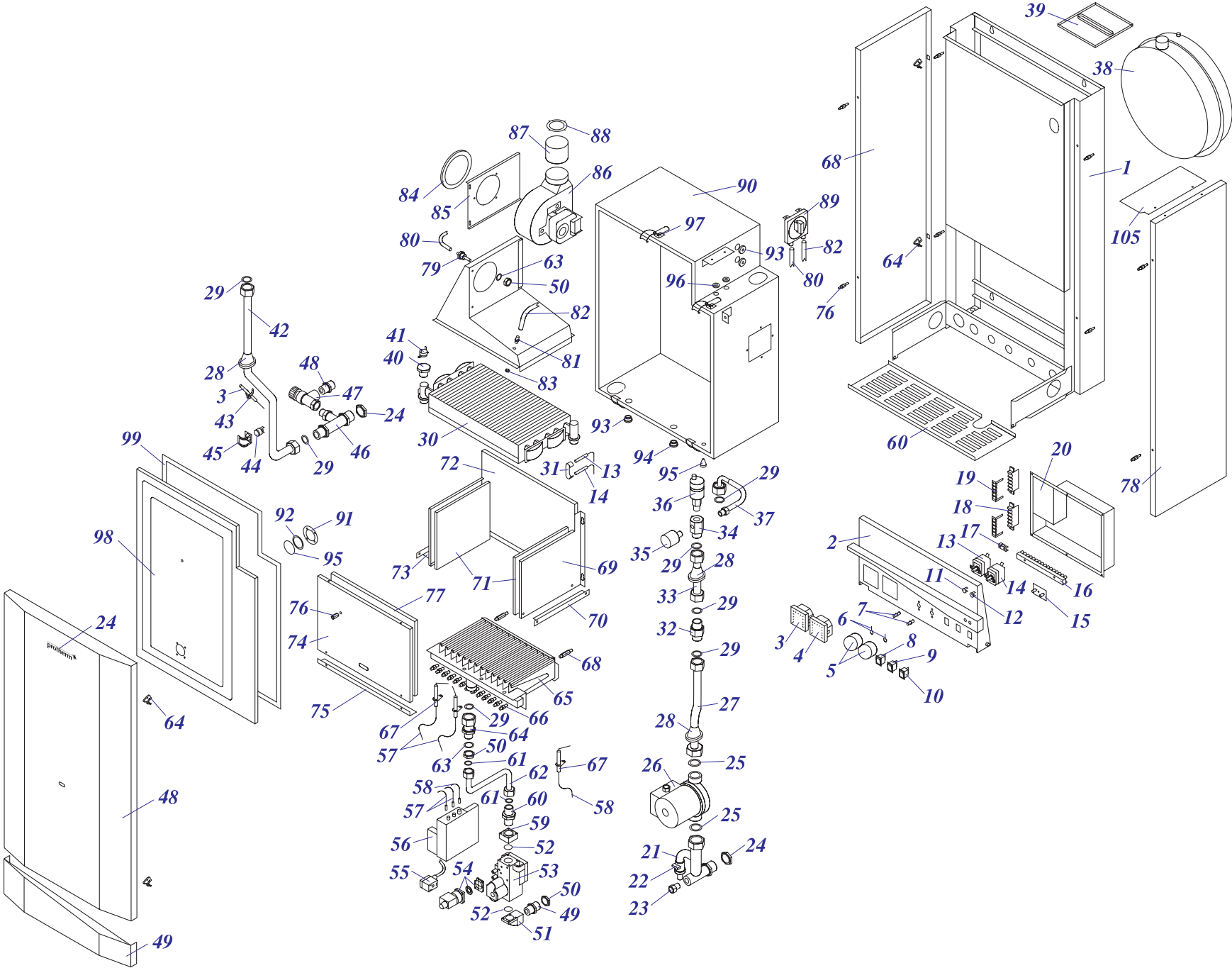
Навесные котлы
