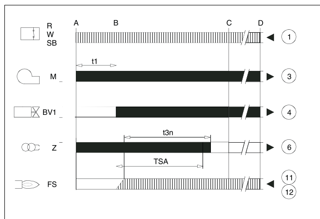
Рис. 9 Выполнение программы автомата горения дизельного топлива
