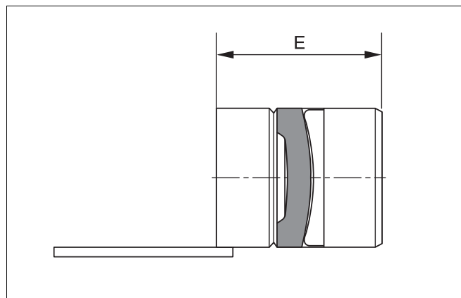
Рис. 5 Жаровой стакан – размер "Е"
