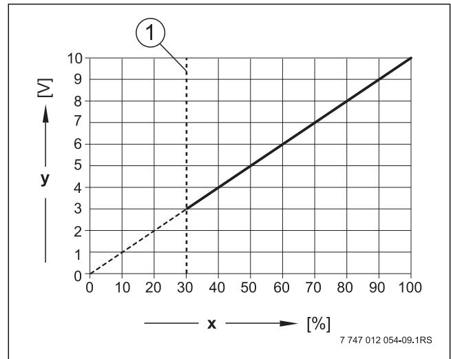
Рис. 27 Клемма U BR сигнал 0–10 В, 0 В = 0%
