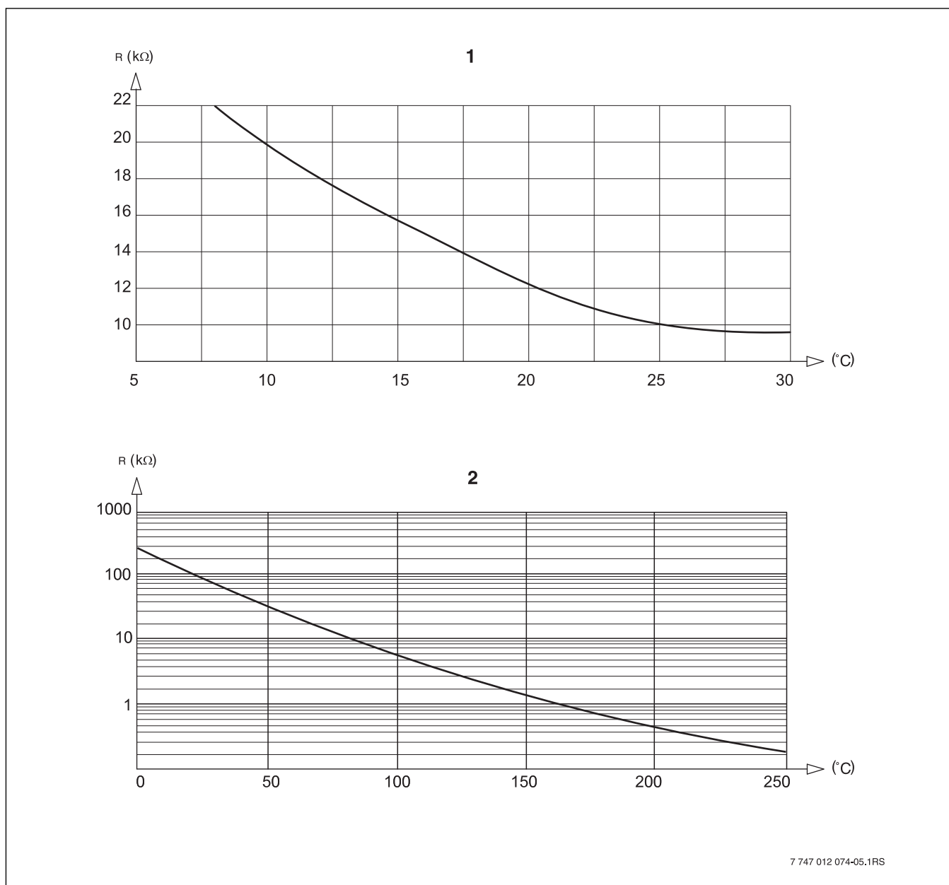
Рис. 87 Датчики комнатной температуры и температуры дымовых газов
