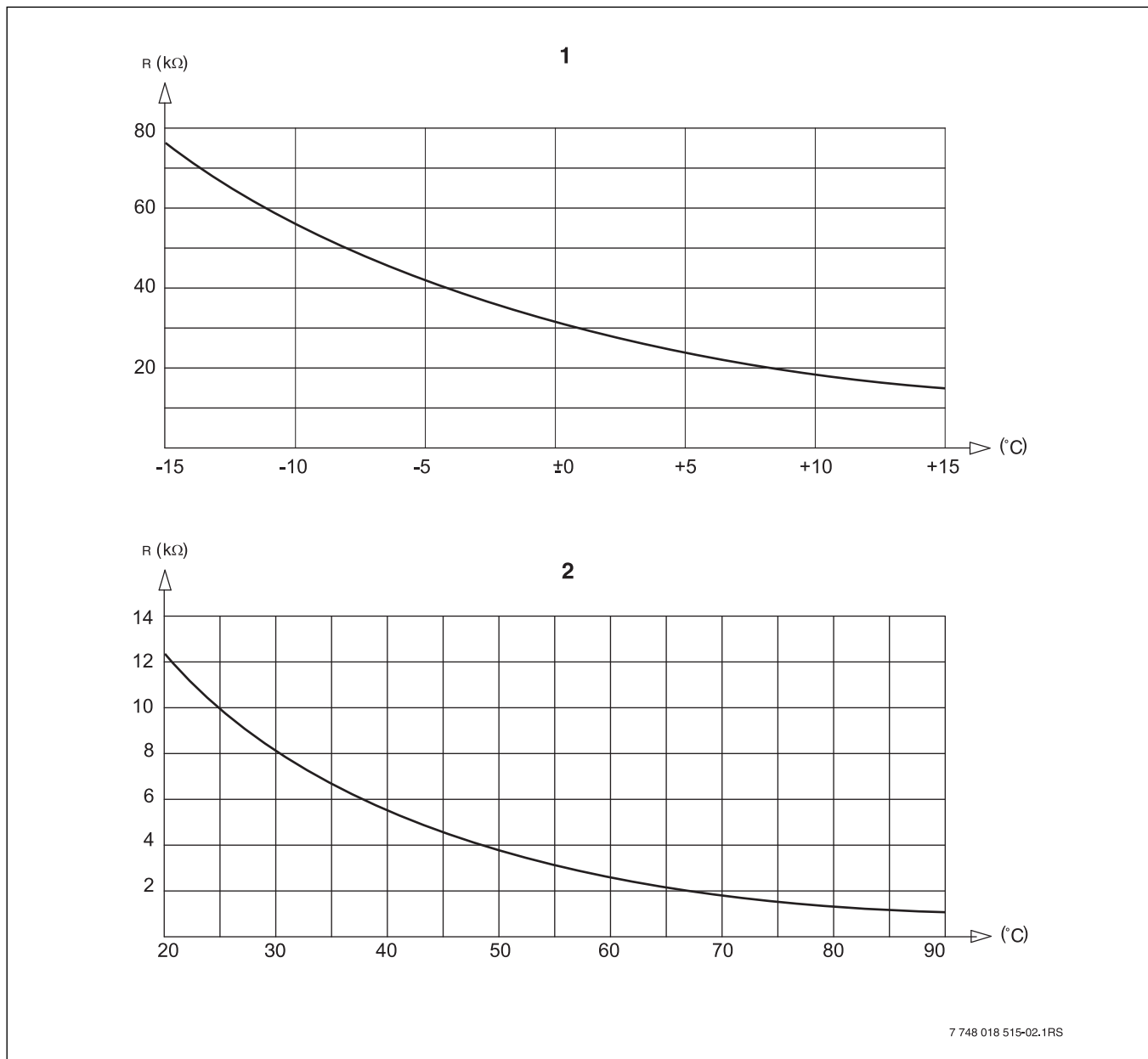
Рис. 86 Датчики наружной температуры, температуры котловой воды, подающей линии, горячей воды
