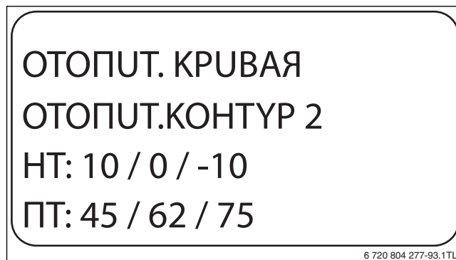
Рис. 76 Отопительная кривая
