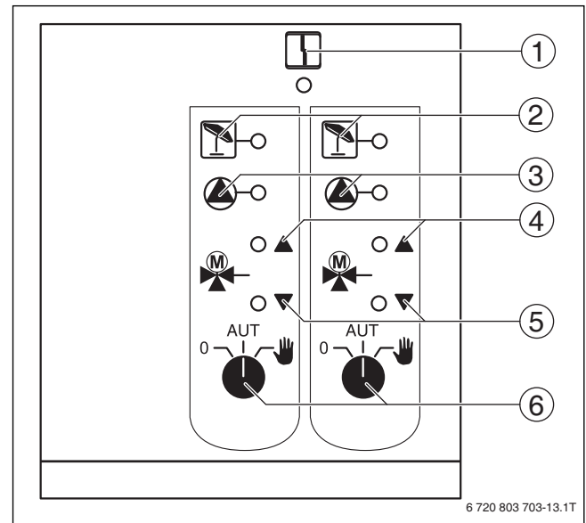
Рис. 13 FM442
