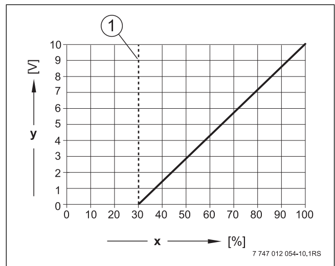
Рис. 28 Клемма U BR сигнал 0–10 В, 0 В = малая нагрузка
