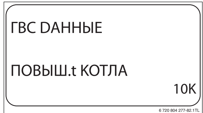
Рис. 66 Повышение температуры котла
