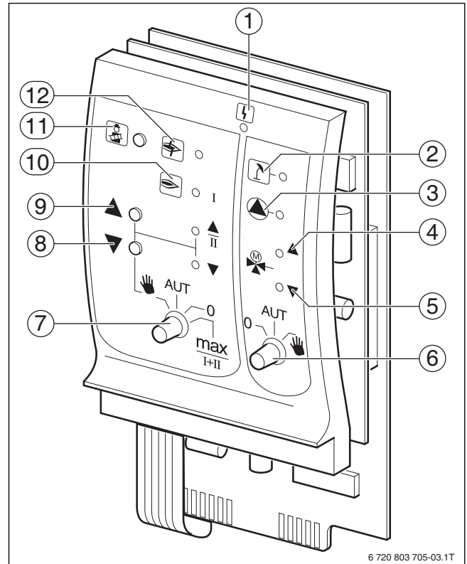
Рис. 11 ZM434
