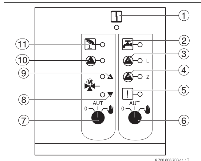
Рис. 12 FM441
