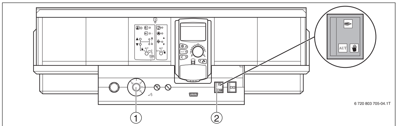
Рис. 14 Проверка STB с переключателем аварийного режима горелки
