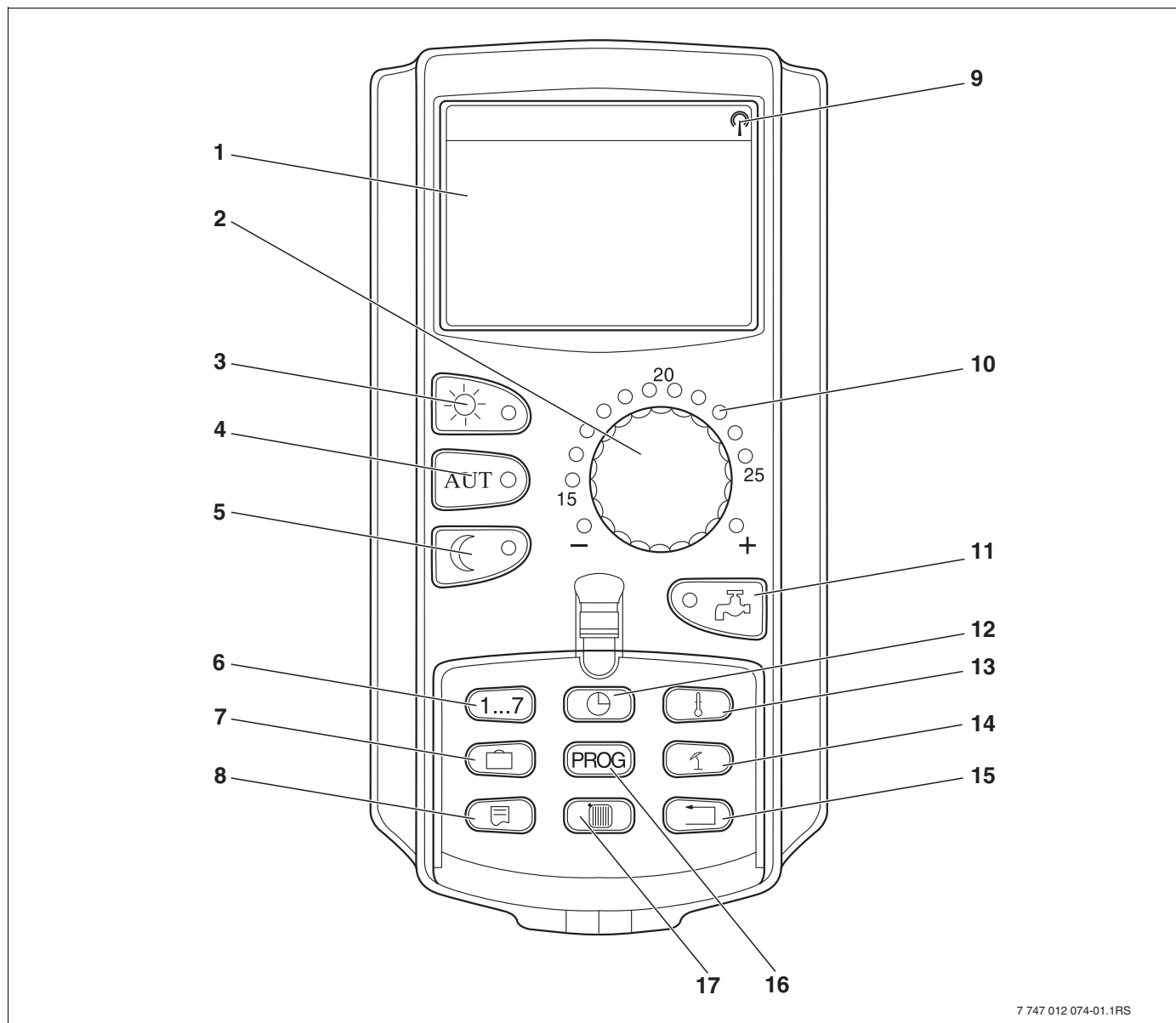
Рис. 8 Пульт управления MEC2
