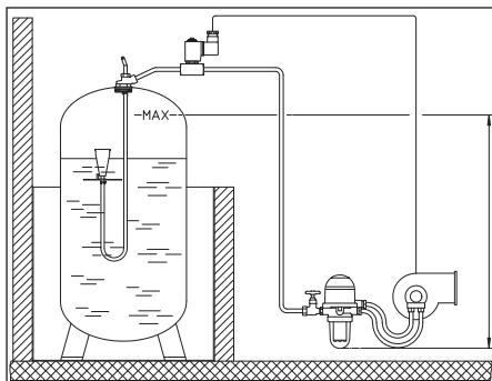
Электромагнитный клапан „Oilstop MV”
