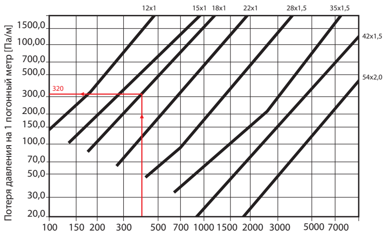
Для одного раствора пропиленгликоля 50:50 Объемный расход [л/ч]
