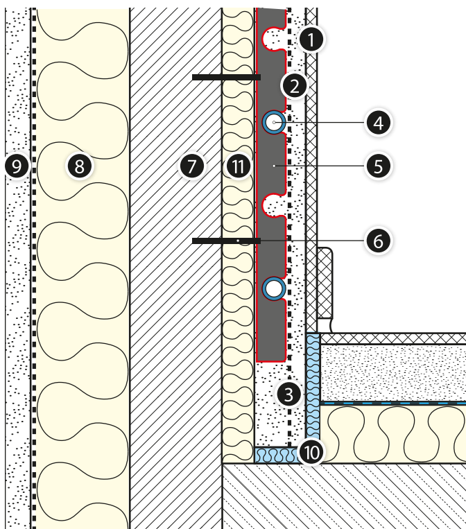
Рис. 32. Конструкция отопления/охлаждения KAN-therm Rail Wall
