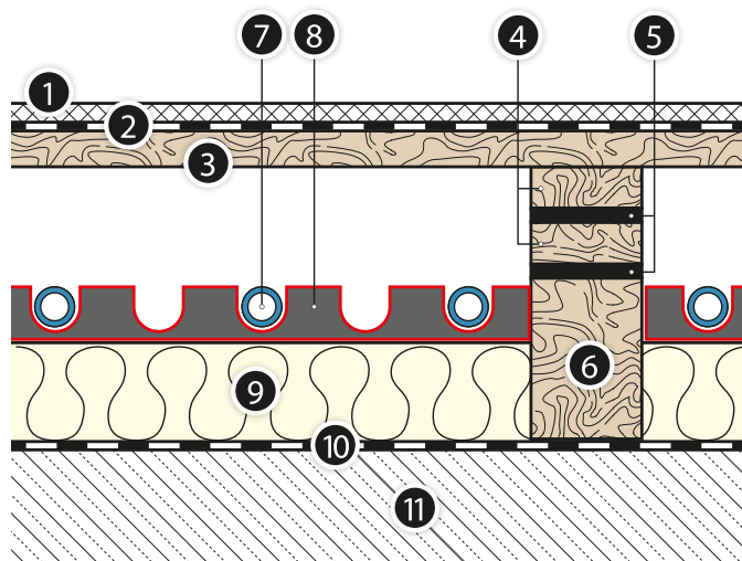
Рис. 38. Конструкция спортивного поверхностно-эластичного пола с системой напольного отопления, выполненного из элементов системы KAN-therm Rail
