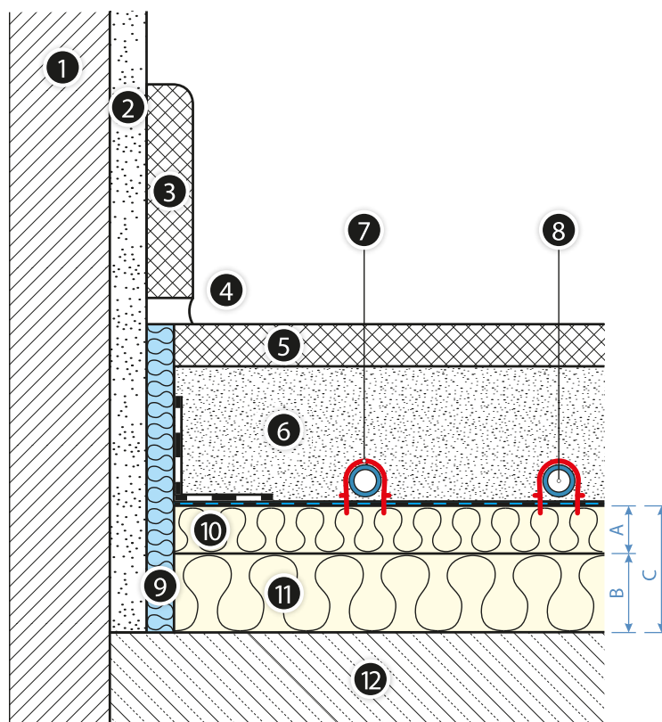
Рис. 22. Напольный отопительный прибор с пенополистирольной плитой KAN-therm Tacker и дополнительной изоляцией на перекрытии над неотапливаемым внутренним помещением, а также перекрытием, контактирующим с наружным воздухом
