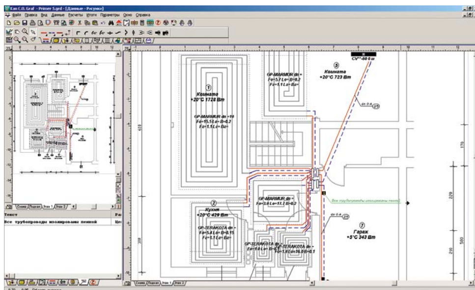
Рис. 81. План этажа с нанесенными напольными отопительными приборами.
