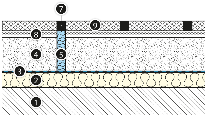
Рис. 15. Выполнение разделительного шва в случае напольного покрытия в виде плитки.
