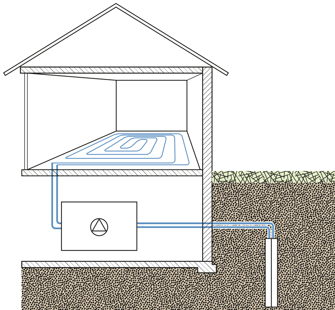
Рис. 2. Подача теплоносителя в систему панельно-лучистого отопления непосредственно от низкотемпературного источника тепла
