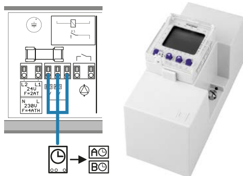
Рис. 76. Схема подключения таймера к клеммной колодке Basic
