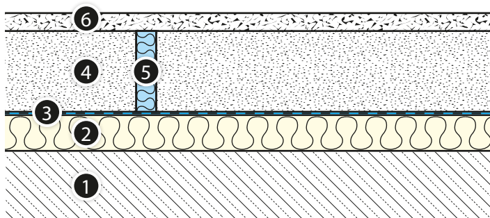
Рис. 14. Выполнение разделительного шва в случае мягкого или „плавающего” напольного покрытия.
