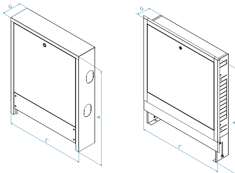
Рис. 52. Размеры монтажных шкафов KAN-therm
