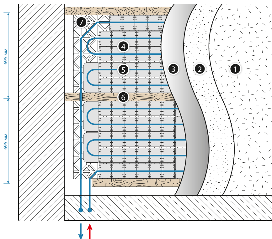
Рис. 35. Конструкция отопления/охлаждения KAN-therm TBS Wall
