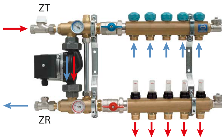
Рис. 60. Коллекторная группа со смесительной системой серии 77A (или 73A) – направления потоков воды
