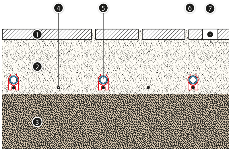
Рис. 40. Подогрев наружных площадок (Система KAN-therm NET)
