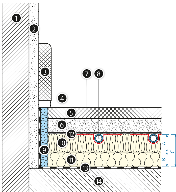
Рис. 30. Напольный отопительный прибор с пенополистирольной плитой KAN-therm TBS и дополнительной изоляцией, а также гидроизоляционным покрытием на полу, на грунте
