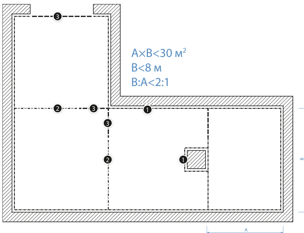
Рис. 17. Принцип выполнения разделительных швов в греющих плитах напольного отопления
