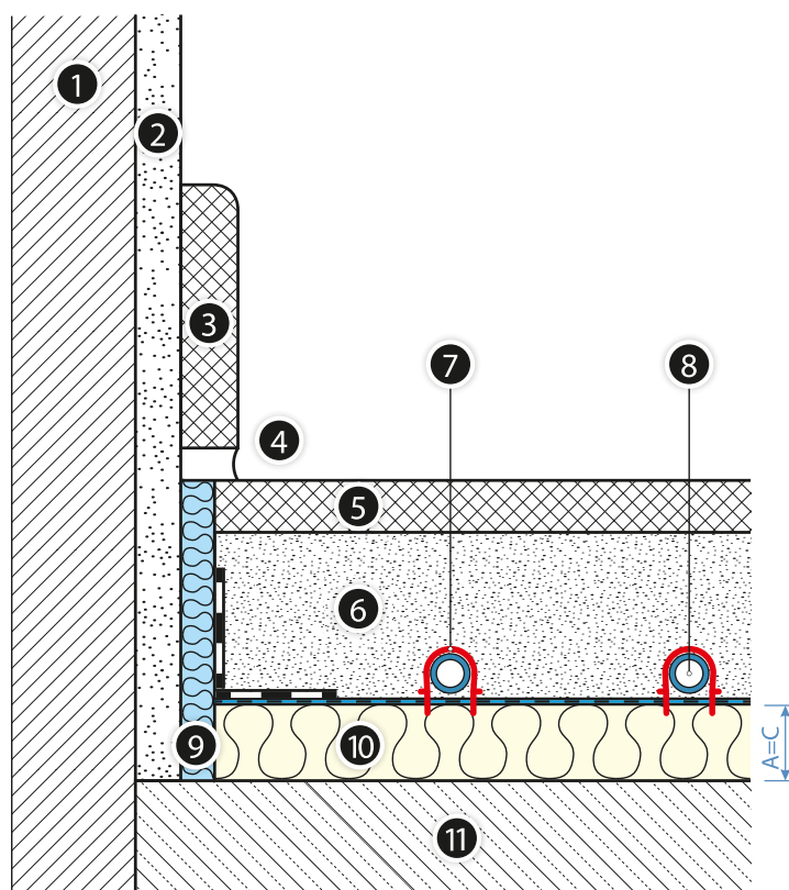
Рис. 21. Напольный отопительный прибор с пенополистирольной плитой KAN-therm Tacker на перекрытии над внутренним помещением
