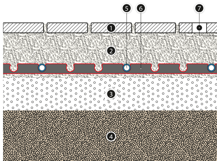
Рис. 39. Подогрев наружных площадок (Система KAN-therm Rail)
