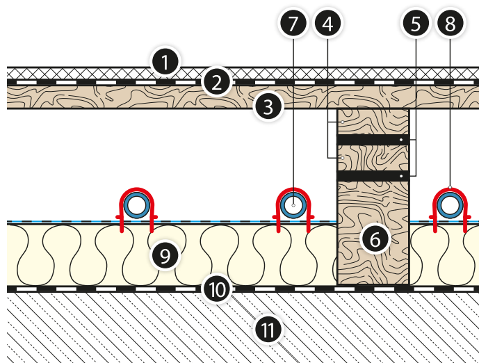
Рис. 37. Конструкция спортивного поверхностно-эластичного пола с системой напольного отопления, выполненного из элементов системы KAN-therm Tacker.
