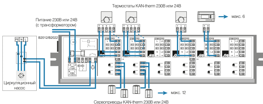
Рис. 68. Конфигурация клеммной колодки Basic 230В или 24В с насосным модулем
