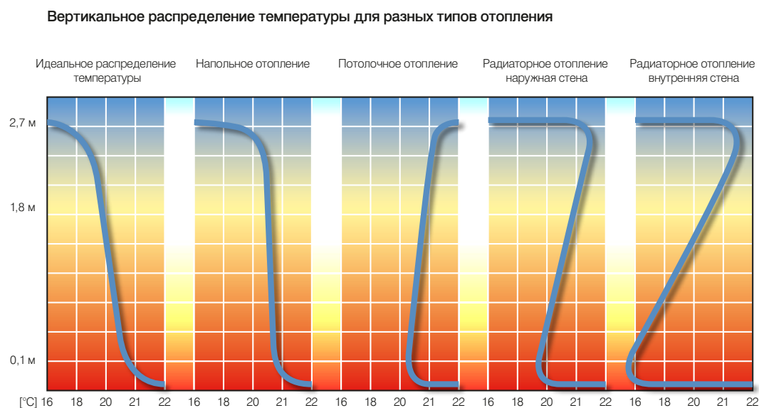
Рис. 1. Вертикальное распределение температуры для разных типов отопления
