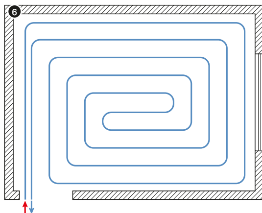
Рис. 6. Контур напольного отопления/охлаждения в форме спирали (улитки).
