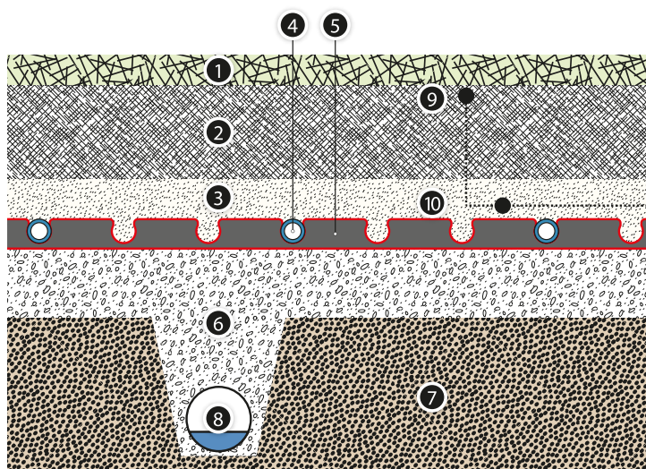
Рис. 44. Футбольное поле – натуральный покров
