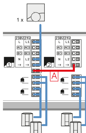
Рис. 69. Подключение 3 или 4 сервоприводов, управляемых одним термостатом
