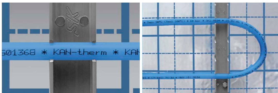
Рис. 33. Крепление труб KAN-therm в стеновом отоплении, выполненным мокрым методом
