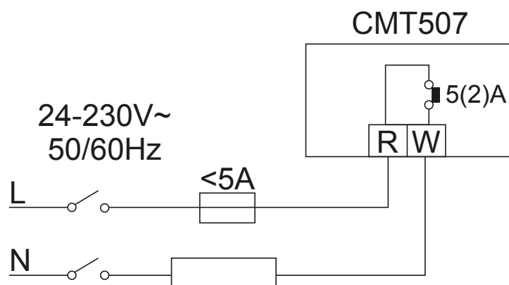
Рис. 65. Схема подключения клемм регулятора с еженедельным программатором 24 – 230 В к клеммной колодке Basic
