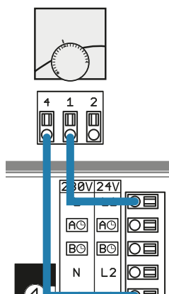
Рис. 62. Схема подключения клемм биметаллического термостата 24 – 230 В (0.6107) к клеммной колодке Basic
