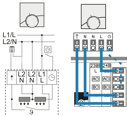
Рис. 63. Схема подключения клемм термостата Basic 230 или 24 В к клеммной колодке Basic (с опцией периодического понижения температуры за счет подключения таймера)
