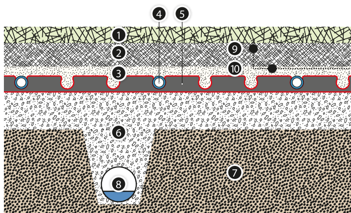
Рис. 45. Футбольное поле – искусственное покрытие
