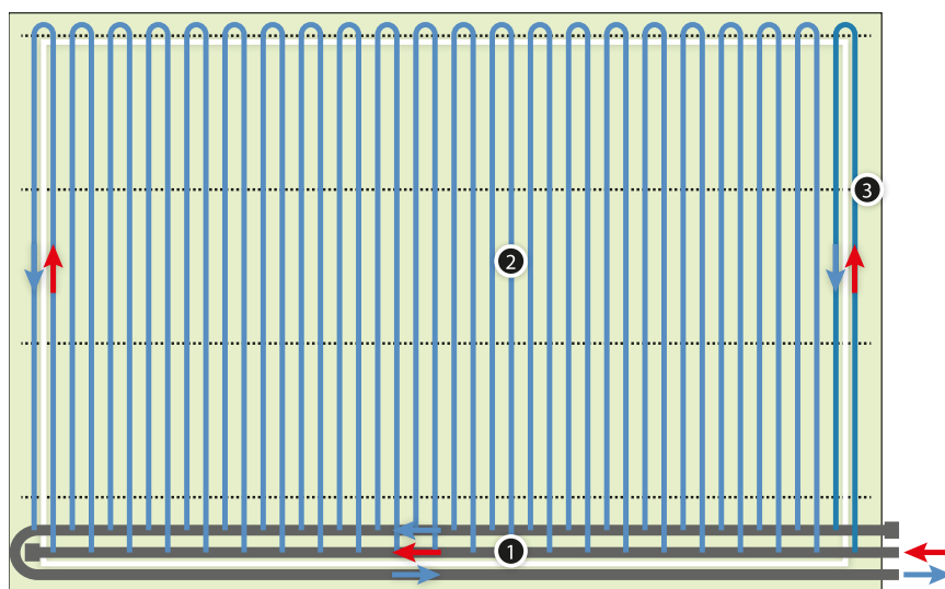
Рис. 42. Схема подогрева футбольного поля системы KAN-therm
