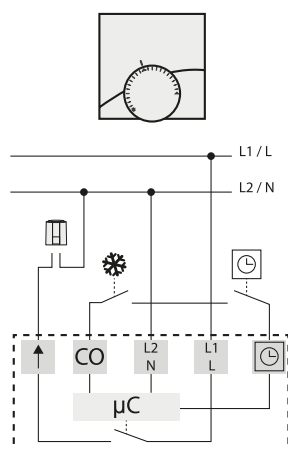
Рис. 64. Схема подключения клемм термостата отопление/охлаждение Basic 230 В или 24 В (с опцией периодического понижения температуры за счет подключения таймера)
