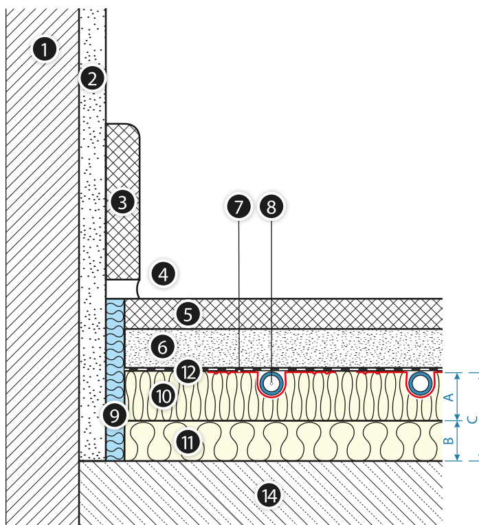
Рис. 29. Напольный отопительный прибор с пенополистирольной плитой KAN-therm TBS и дополнительной изоляцией на перекрытии над внутренним помещением, а также перекрытии, контактирующим с наружным воздухом
