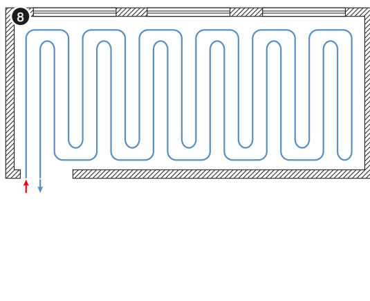
Рис. 8. Контур напольного отопления/охлаждения двойной меандр.
