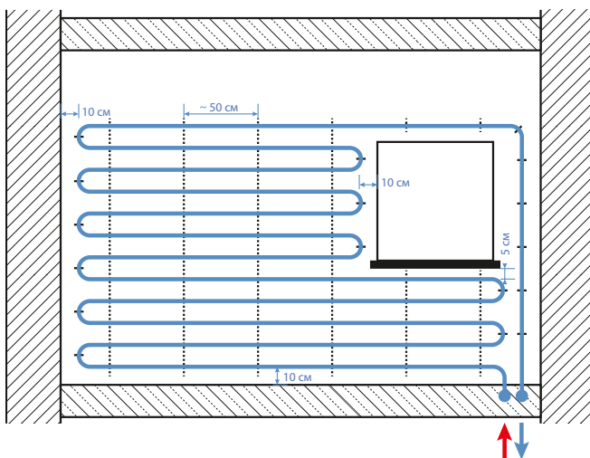
Рис. 31. Монтажные расстояния в стеновом отоплении
