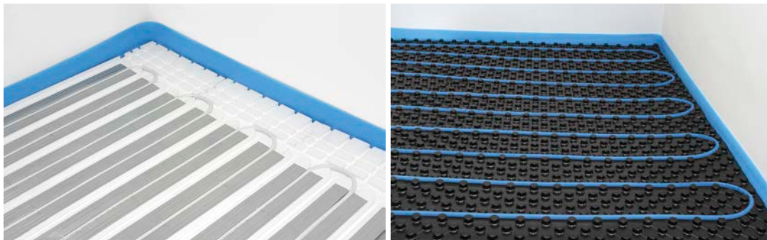
Рис. 12. Примеры монтажа краевой ленты в напольном отоплении KAN-therm.
