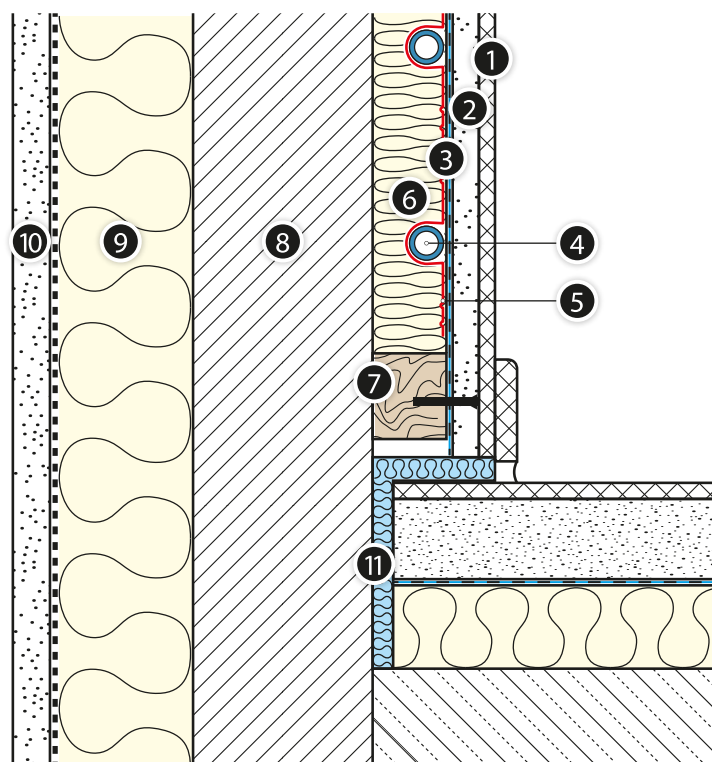
Рис. 34. Конструкция отопления/охлаждения KAN-therm TBS Wall
