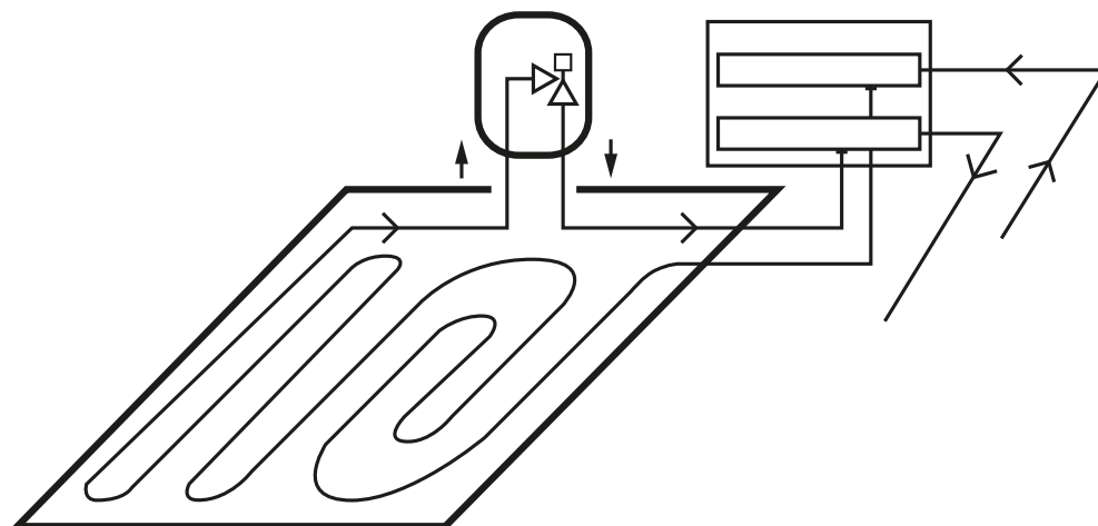
Рис. 77. Схема работы – комплект расположен на обратке.
