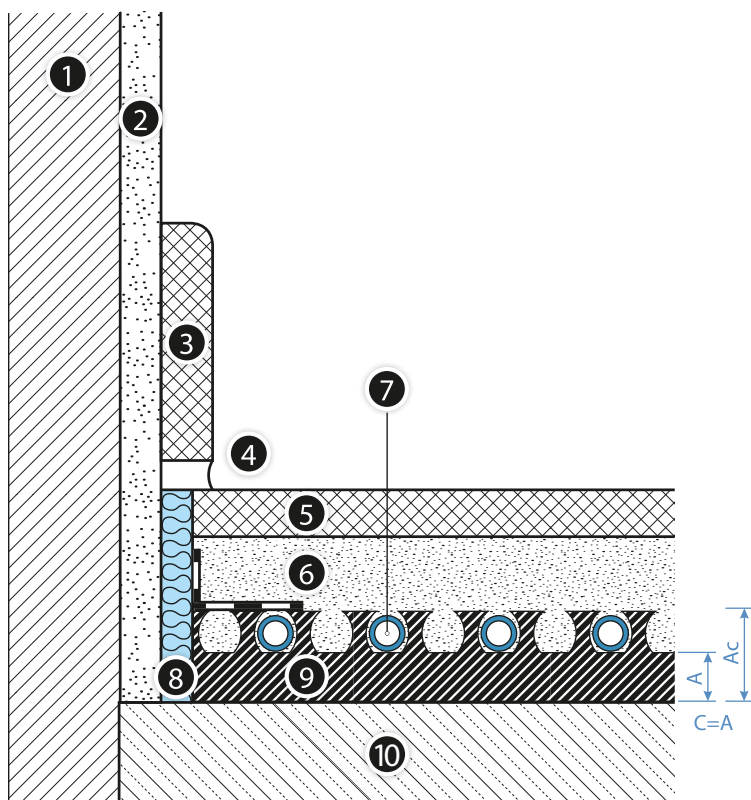
Рис. 25. Напольный отопительный прибор с системной плитой KAN-therm Profil на перекрытии над внутренним помещением
