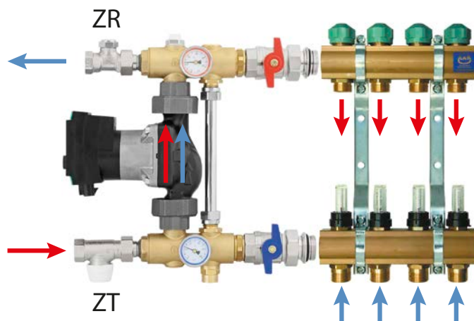
Рис. 61. Насосная группа K-803003 (или K-803000, K-803001) с коллекторной группой 75A (или 71A, 55A, 51A) – направления потоков воды
