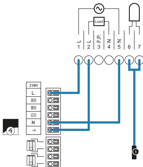
Рис. 66. Схема подключения клемм терморегулятора с еженедельным программатором TH232-AF
