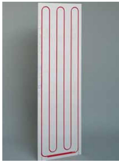
3 Рис. 22: KES- панель большая ШУ104 Длина панели: 200 см Ширина панели: 62 см Толщина панели: 18 мм Шаг укладки: 104 мм Вес: 24,18 кг Длина уложенной трубы: 12,4 м
