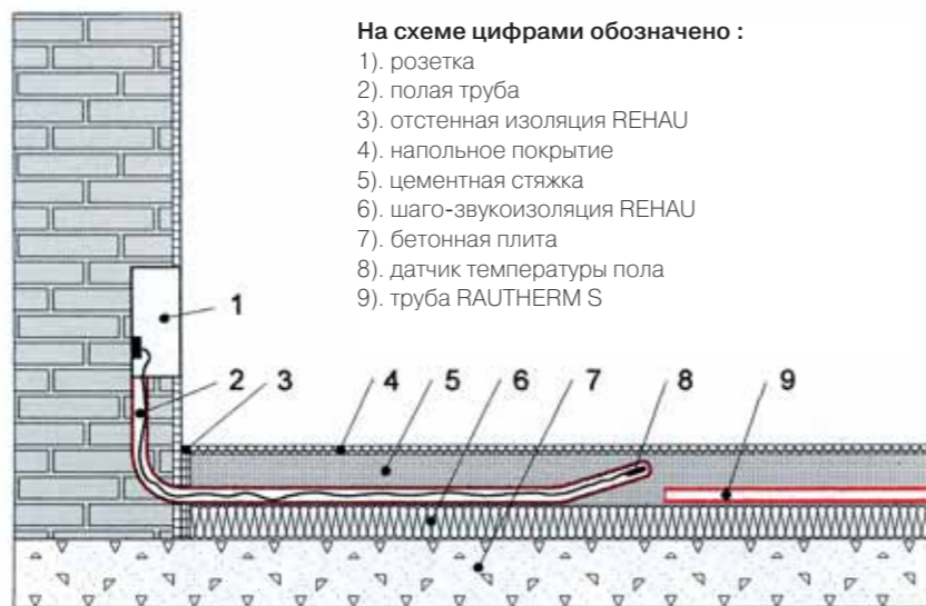
1 Рис. 97: Монтаж датчика температуры пола
