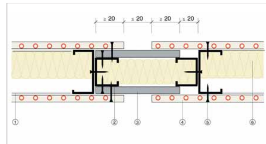
3 Рис. 33: Пример схемы деформационных и компенсационных швов
