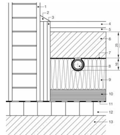
"Сухая" система REHAU с уложенной трубой RAUTHERM S
