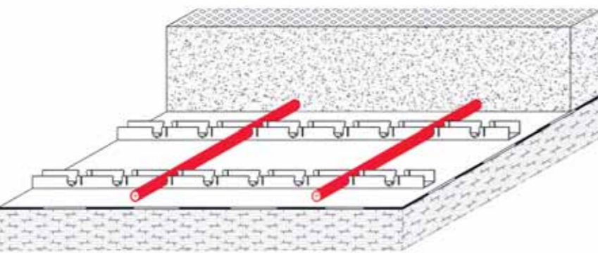
6 Рис. 10: Бетонная плита, армированная стальными волокнами; специальная конструкция: отопительные трубы смонтированы на фиксирующих шинах
