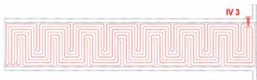
6 Рис. 28: Обогрев пандуса
