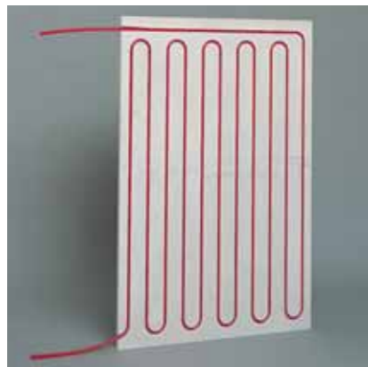
3 Рис. 24: KES- панель поперечная ШУ 75 Длина панели: 83 см Ширина панели: 125 см Толщина панели: 18 мм Шаг укладки: 75 мм Вес: 20,23 кг Длина уложенной трубы: 14,4 м
