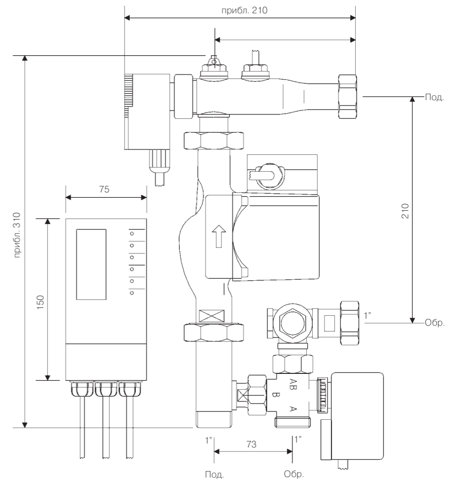
1 Рис. 71 : Размеры терморегулирующей станции TRS-T
