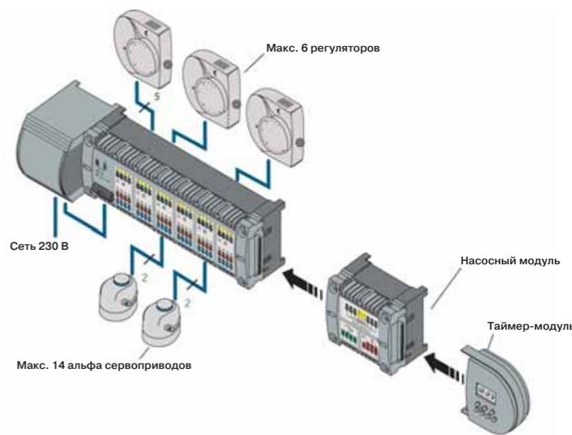
1 Рис. 72: Схема подключения компонентов прибора RAUMATIC M
