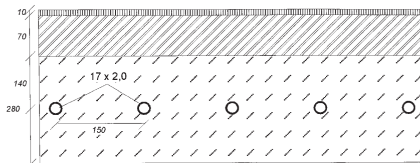
5 Рис. 37: Конструкция плиты перекрытия ВКТ в разрезе
