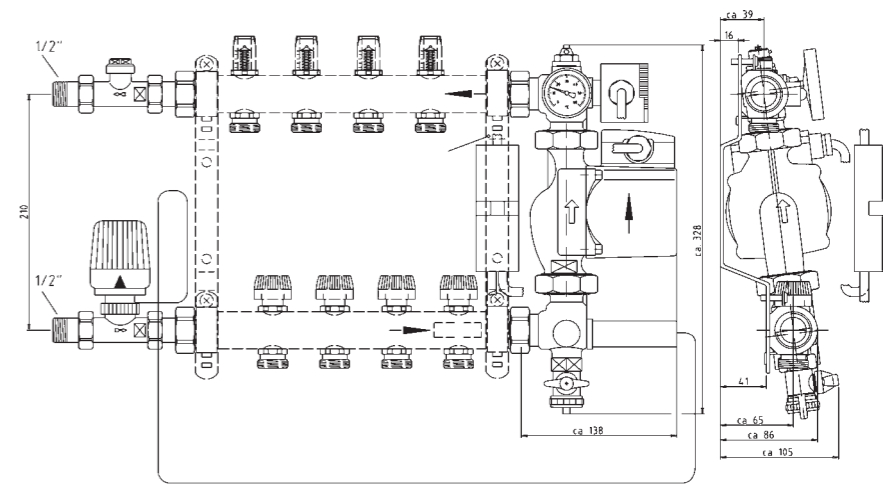
1 Рис. 68: Комплект температурного регулирования с постоянными параметрами
