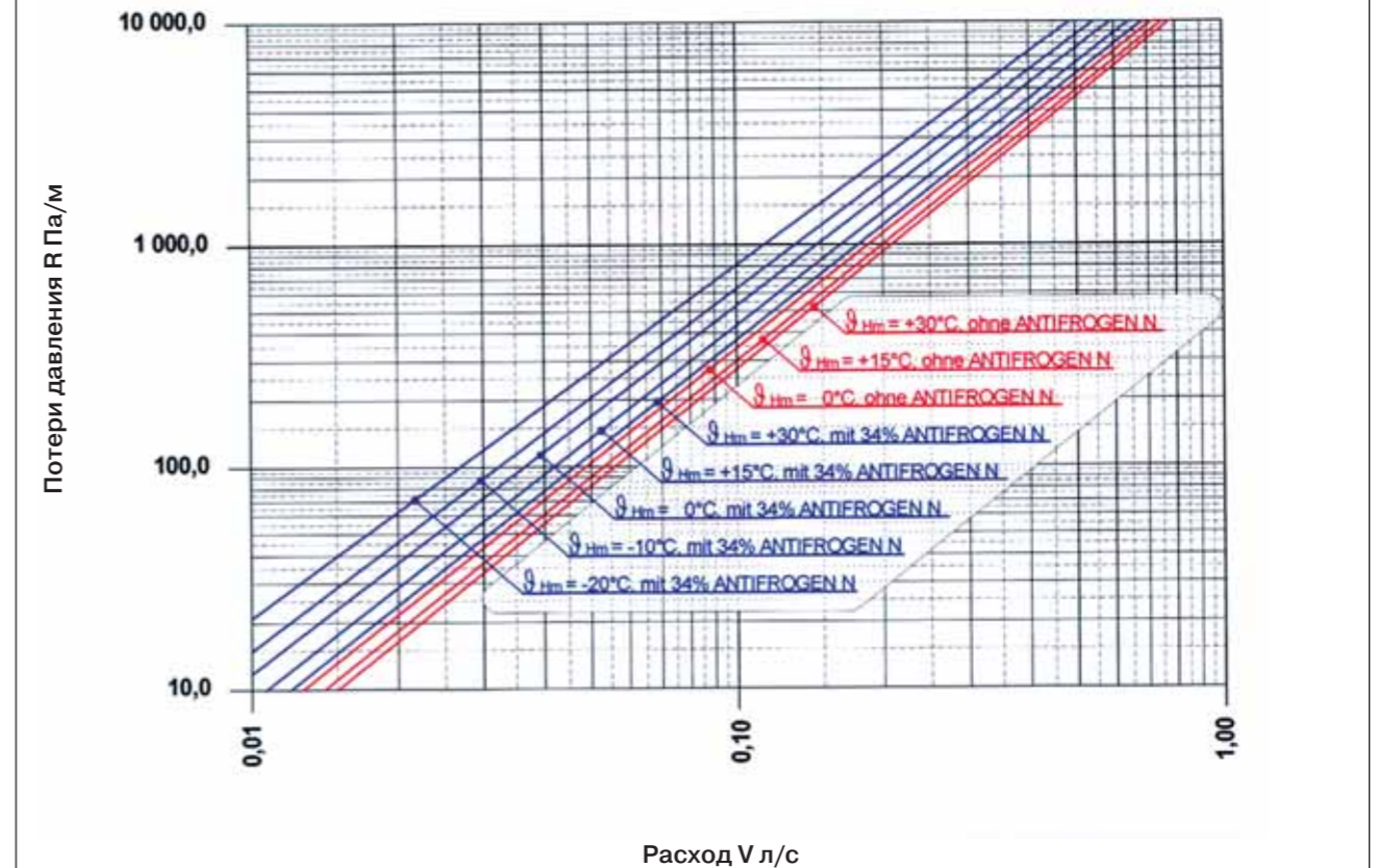
Диаграмма потерь давления для труб RAUTHERM S 20x2,0
