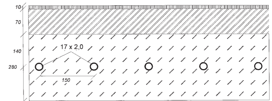
5 Рис. 43: Конструкция плиты перекрытия ВКТ в разрезе
