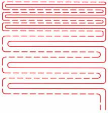
1 Рис. 81: Метод укладки двойной змеевик с более плотной укладкой в граничной зоне
