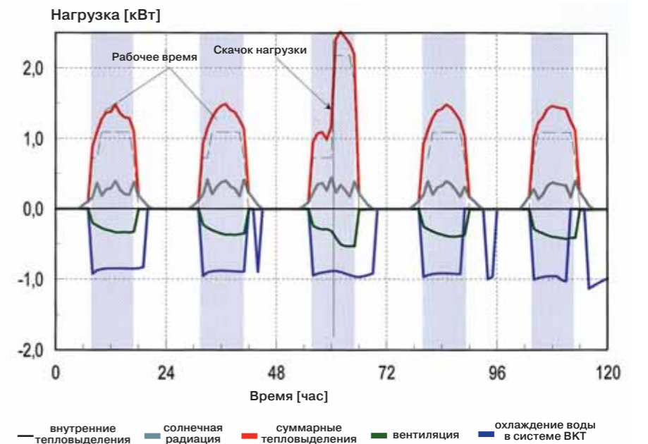
5 Рис. 39: График нагрузок в режиме охлаждения/Вариант А
