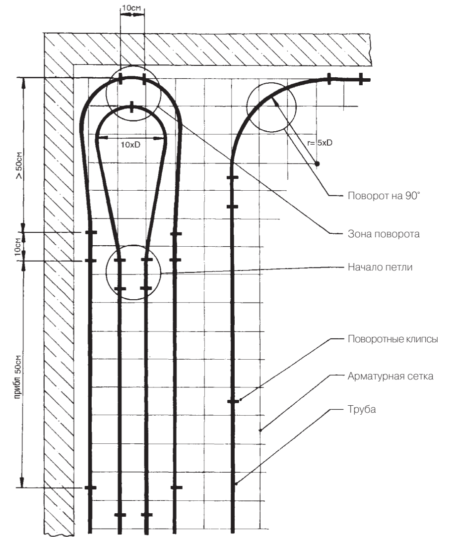
1 Рис. 33: Разворот и поворот труб в контуре
