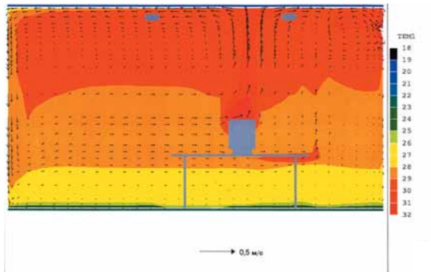
5 Рис. 45: Вертикальный разрез по сечению X2. Моделирование воздушных потоков/Режим охлаждения
