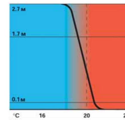
Идеальное распределение температур по высоте помещения
