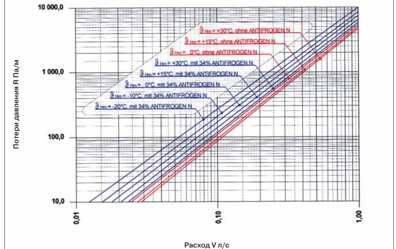
Диаграмма потерь давления для труб Rohr RAUTHERM S 20x2,0
