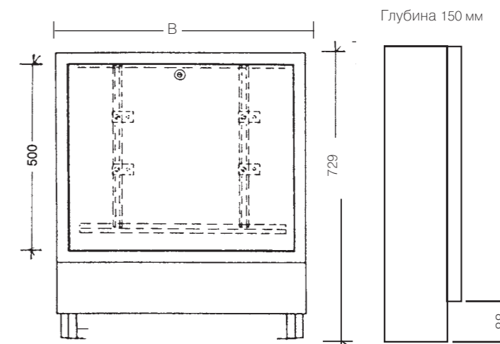
1 Рис. 58: Присоединительные размеры приставного распределительного шкафа
