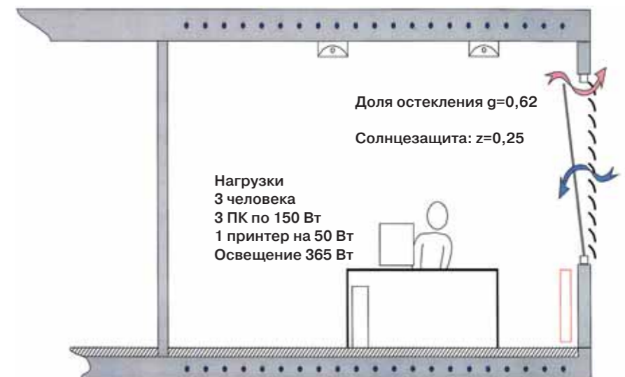
5 Рис. 42: Поперечный разрез по представительному помещению
