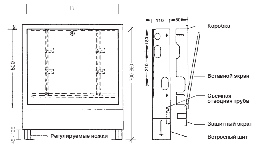
1 Рис 57: Присоединительные размеры встроенного распределительного шкафа
