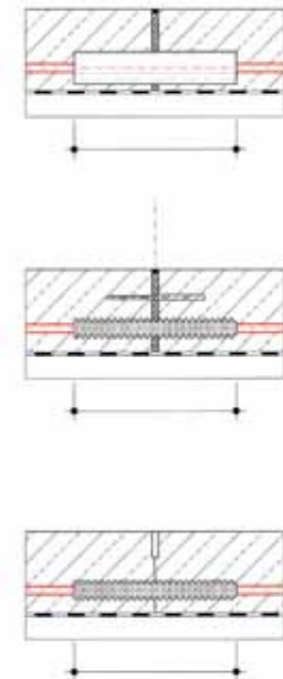
6 Рис. 11 Защита отопительных труб при пересечении ими температурного шва
