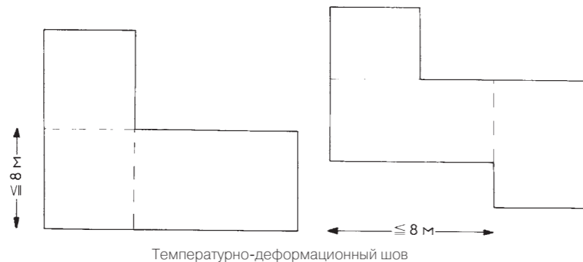
1 Рис. 88: Устройство швов
