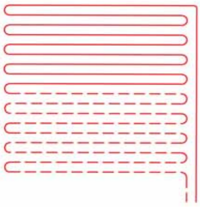
1 Рис. 83: Метод укладки змеевик
