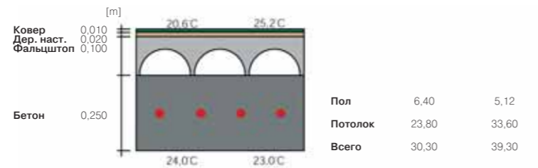
5 Рис. 49: Конструкция плиты 4
