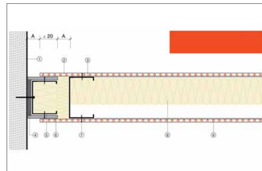
3 Рис. 35: Пример схемы скользящих швов примыкания фасадов
