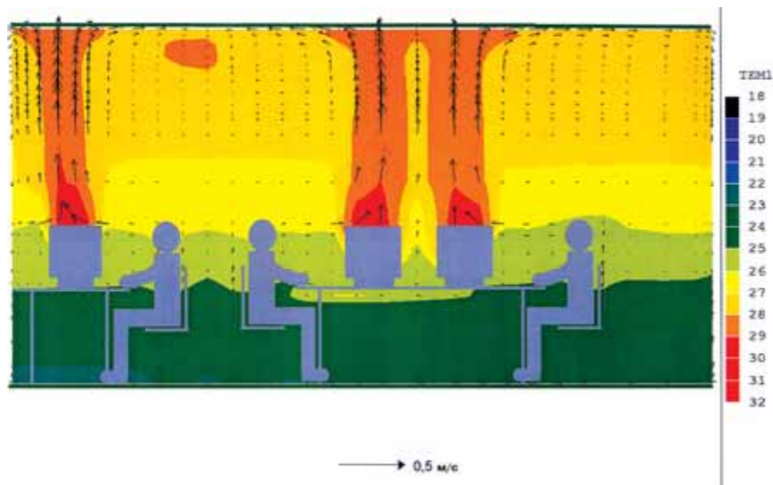
5 Рис. 40: Разрез по сечению Y. Моделирование воздушных потоков/Режим охлаждения
