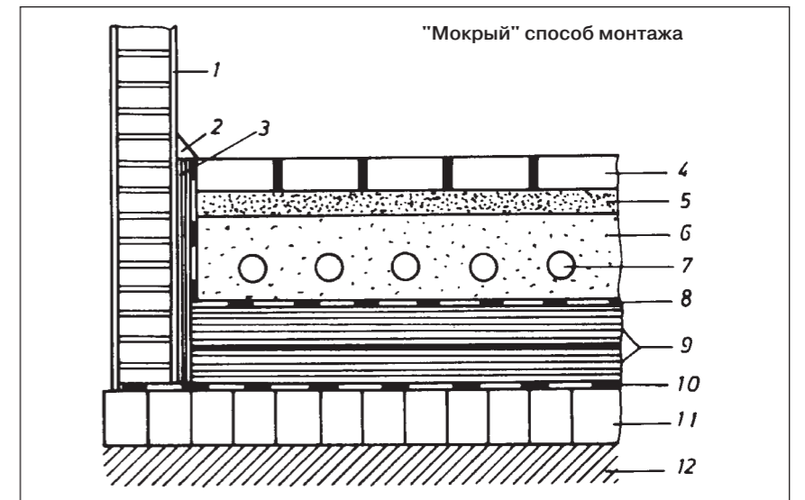
1 Рис. 76: Конструкция пола при "мокром" способе монтажа.
