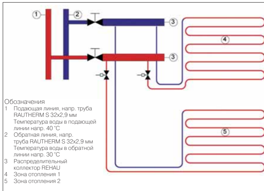
4 Рис. 2: Схематическое представление коллекторного присоединения зон отопления
