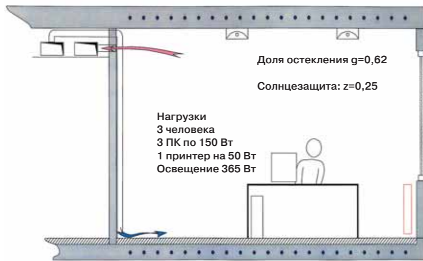
5 Рис. 36: Поперечный разрез представительного помещения/Вариант А
