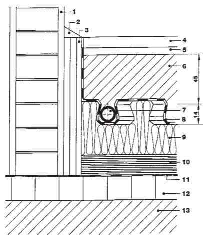
1 Рис. 100: Система напольного отопления REHAU RAUFIX с использованием фиксирующих шин, в разрезе
