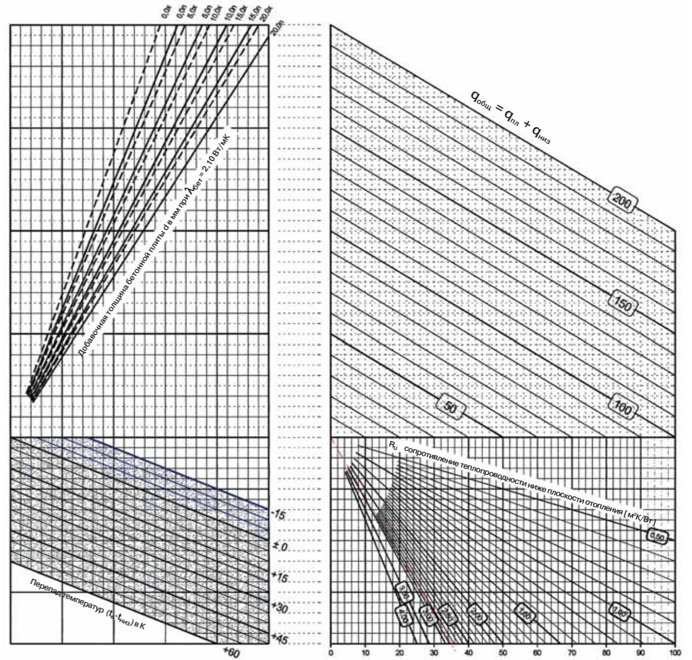
q_{низ} удельные потери тепла плиты вниз [Вт/м²]
