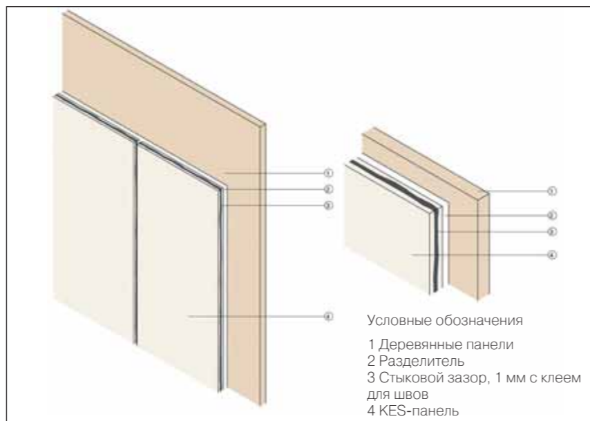
3 Рис. 30: KES-панель на деревянной конструкции.
