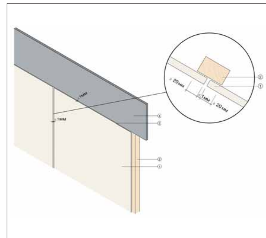
3 Рис.34: Пример схемы стыковых швов
