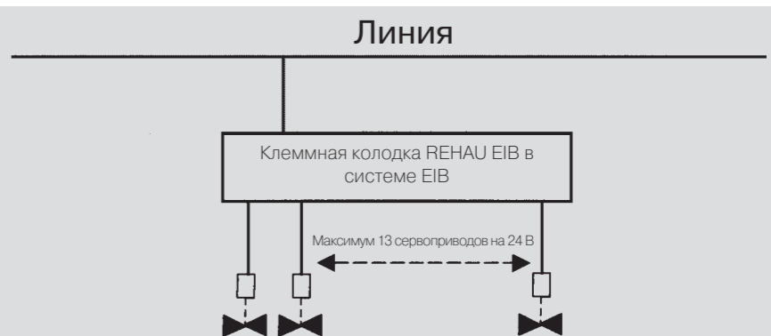
1 Рис. 73: Клеммная колодка EIB REHAU с проводом для BUS-разъема
