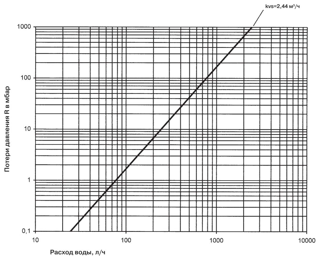
2 Рис. 4: Диаграмма расхода воды для вентиля на обратной гребенке -НКВ
