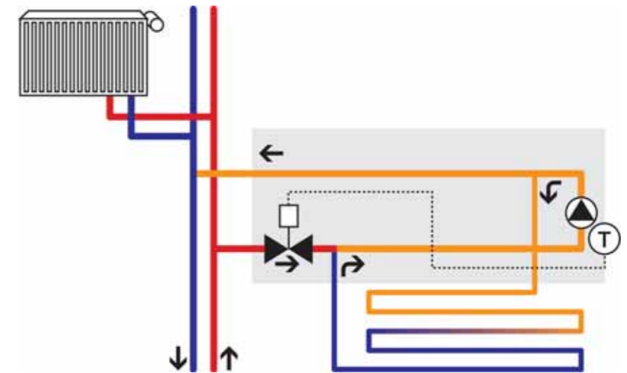
1 Рис. 69: Схема подключения
