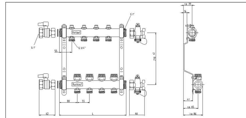
1 Рис. 54: Присоединительные размеры распределительного коллектора НКВ
