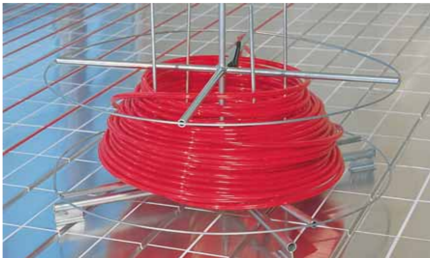
1 Рис. 57: Устройство для размотки труб REHAU
