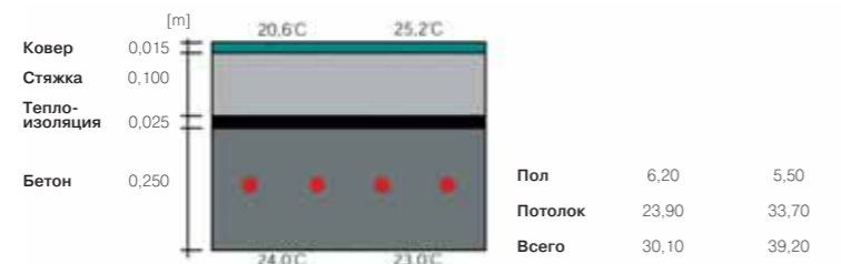
5 Рис. 47: Конструкция плиты 2
