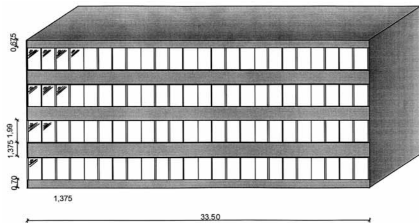
5 Рис. 33: Представительное здание
