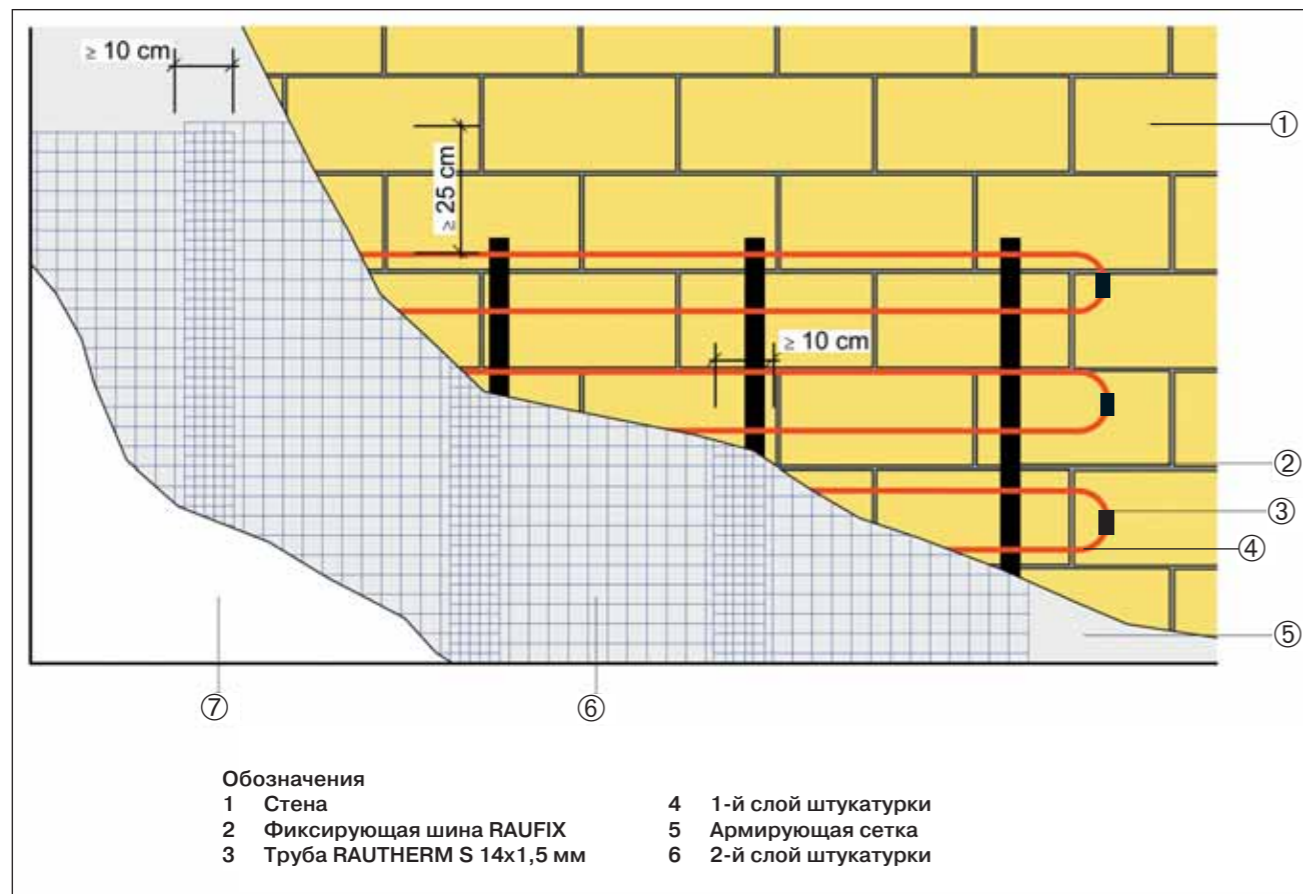
3 Рис. 19: Монтаж фрагмента системы настенного отопления
