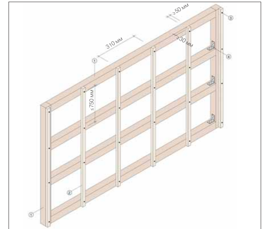
3 Рис. 28: Указания по исполнению каркасных конструкций
