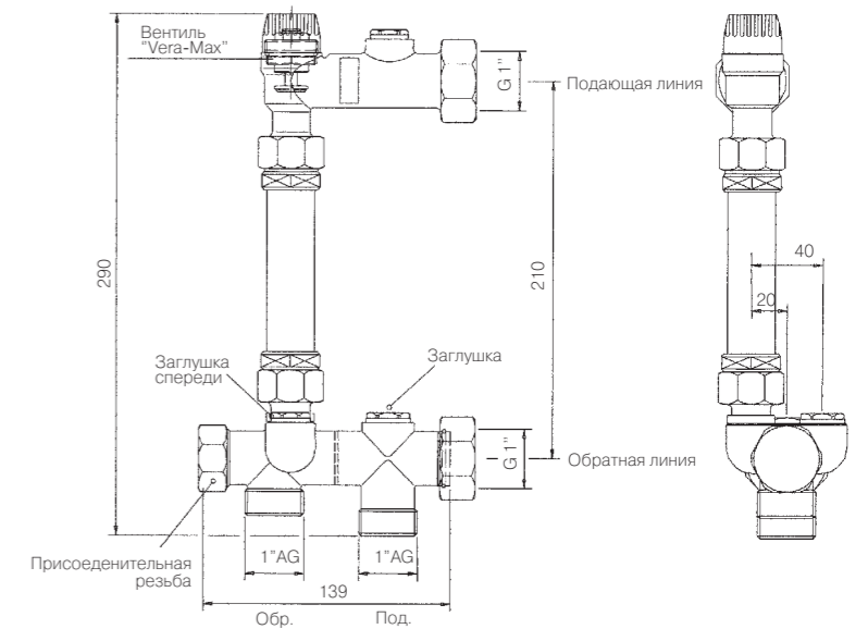
1 Рис. 61: Размеры комплекта для установки теплосчетчика REHAU
