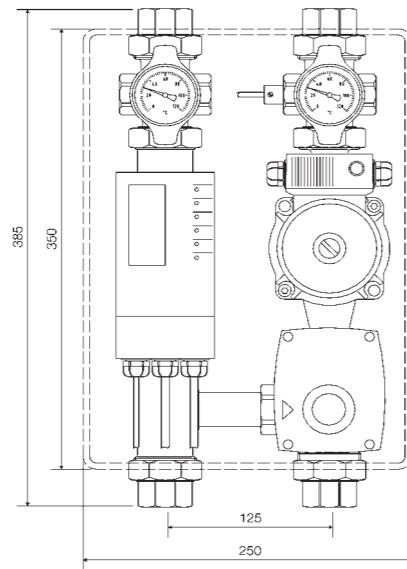
1 Рис. 65: Терморегулирующая станция TRS-20
