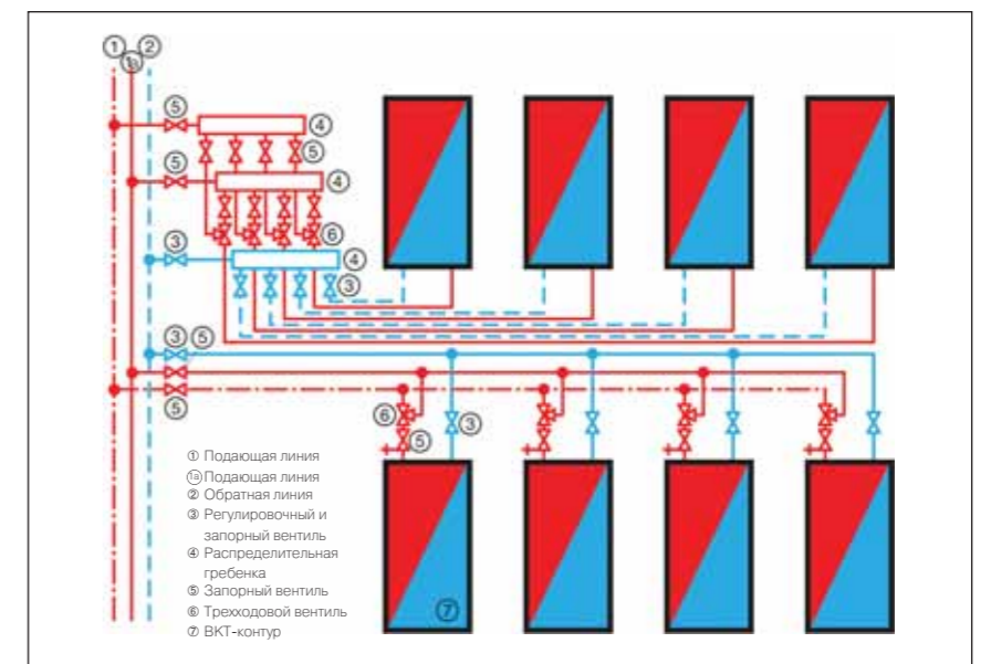
5 Рис. 52: Схематичное представление трехтрубной системы
