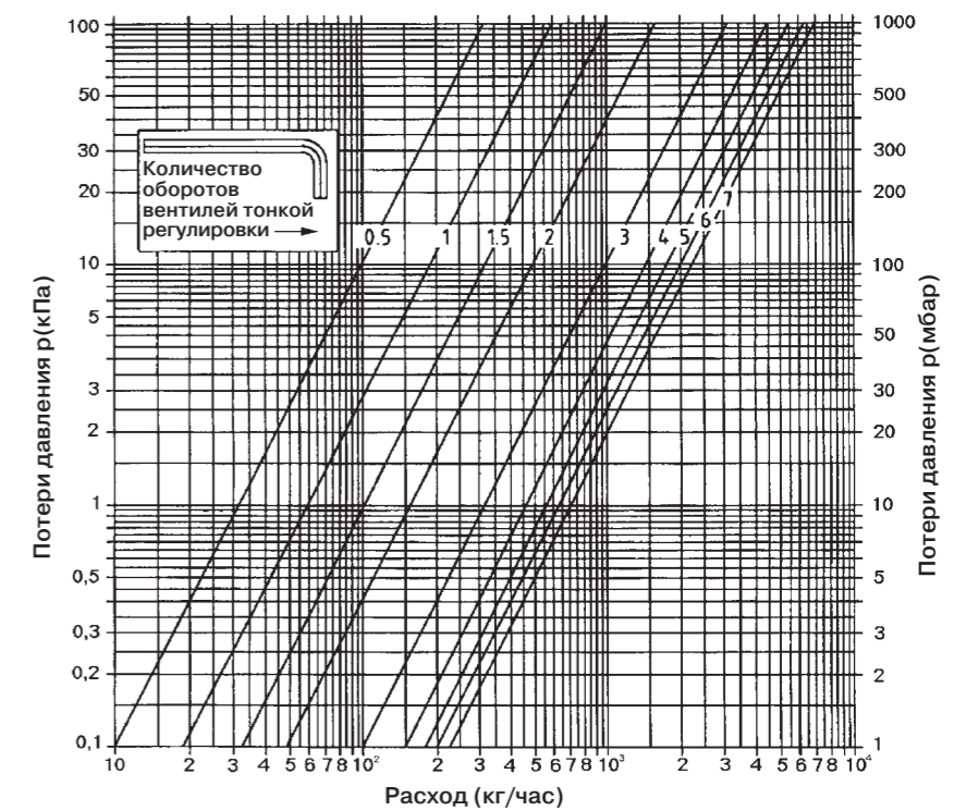
1 Рис. 62: Диаграмма для определения величины установочной регулировки расхода вентиля тонкой регулировки комплекта для установки теплосчетчика.
