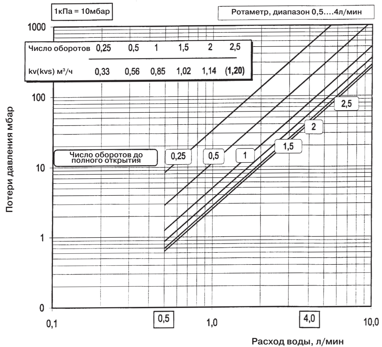
2 Рис. 6: Характеристики вентиля тонкой регулировки на распределительном коллекторе НКV-D
