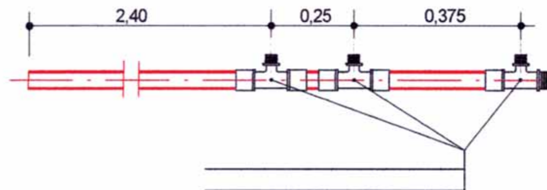
6 Рис. 23: Распределительный коллектор REHAU
