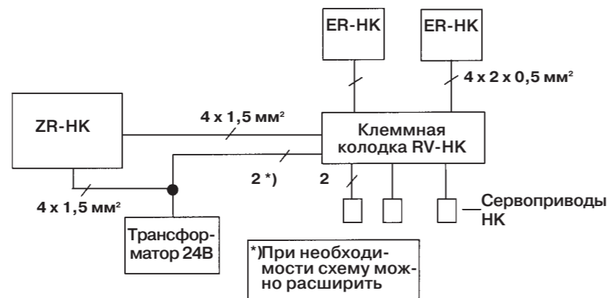
1 Рис. 96: Принципиальная схема подсоединения к клеммной колодке RV-НК
