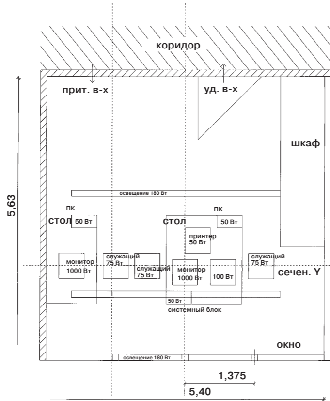
5 Рис. 34: План представительного помещения
