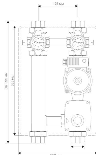
1 Рис.67: Смесительный узел PMG-25
