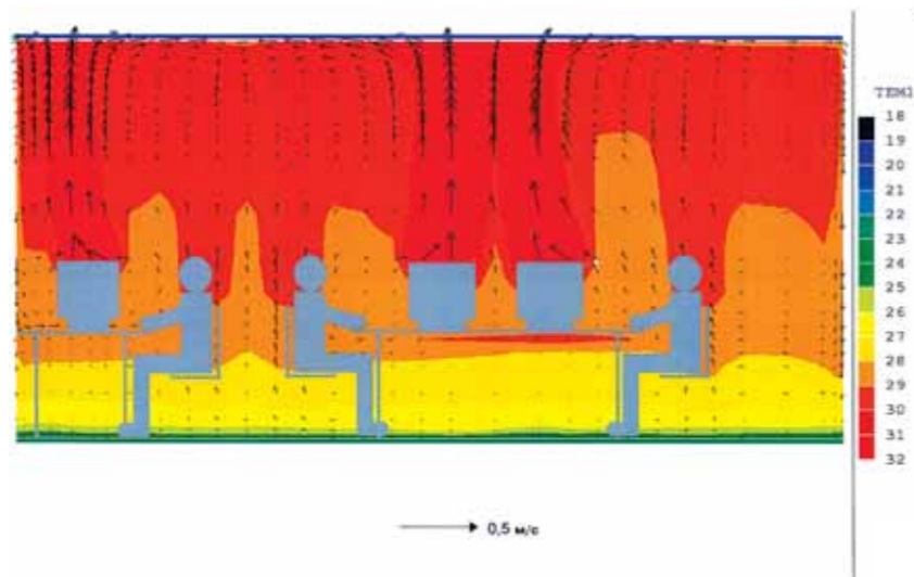
5 Рис. 44: Вертикальный разрез по сечению Y. Моделирование воздушных потоков/Режим охлаждения.
