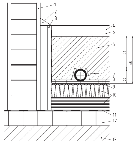
Монтаж на фиксирующих шинах RAUFIX REHAU с уложенной в них трубой RAUTHERM-S в разрезе
