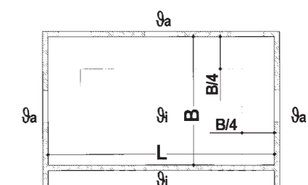
6 Рис. 13: Разбивка зон
