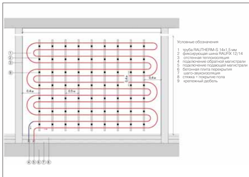
3 Рис. 16: Схематичное изображение системы настенного отопления REHAU с укладкой труб двойным змеевиком при "мокрый" способе монтажа
