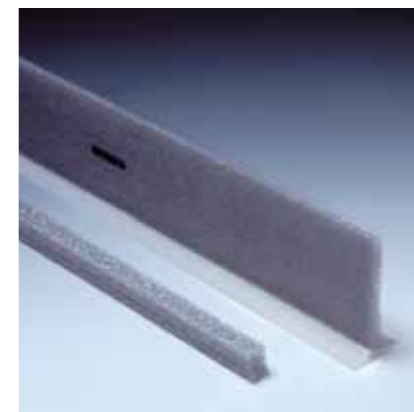
1 Рис. 42: Профиль для деформационного шва и дополнительный профиль REHAU
