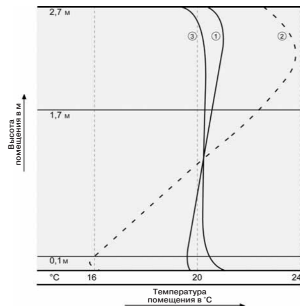
3 Рис. 3: Сравнение кривой распределения температур по высоте помещения при системе настенного отопления RENAУ 1, традиционной системе отопления 2 с идеальной кривой распределения температур по высоте помещения 3
