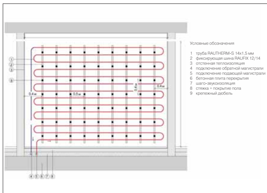
3 Рис. 15 Схематичное изображение системы настенного отопления REHAU с укладкой труб змеевиком при "мокрый" способе монтажа
