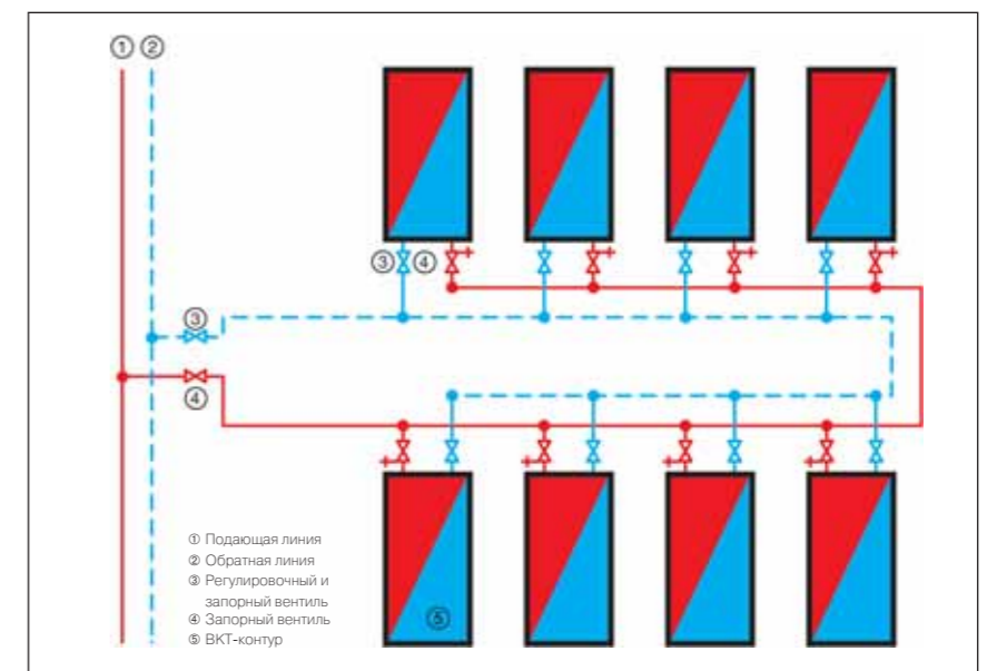
5 Рис. 51: Схематичное представление двухтрубной системы
