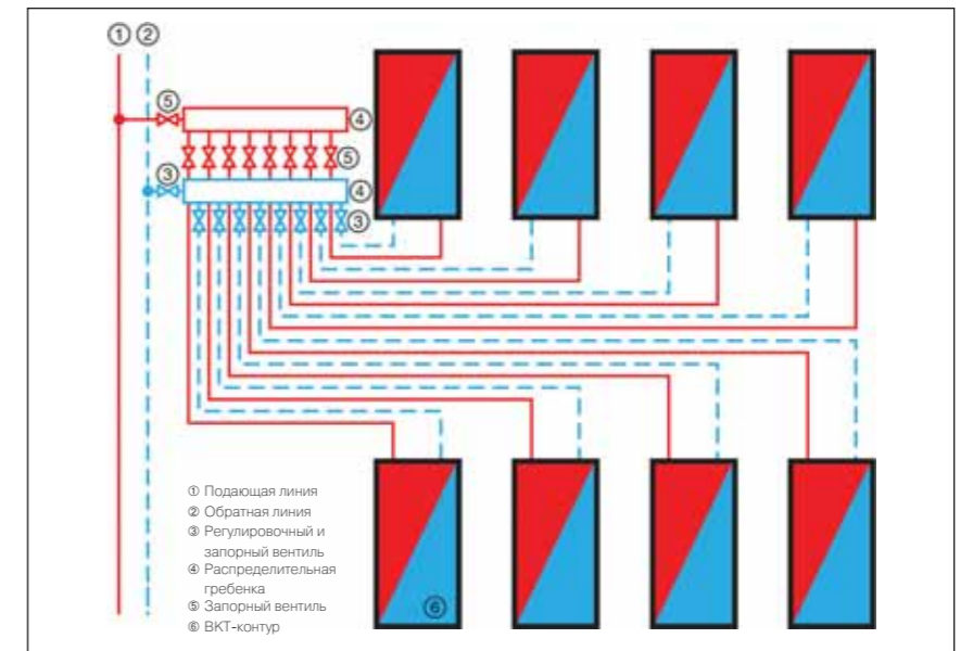
5 Рис. 50: Схема подключения к коллектору
