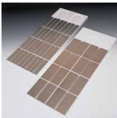
1 Рис. 35: Теплоизоляционные маты REHAU под шаг укладки 12,5/25 см с поворотными элементами REHAU
