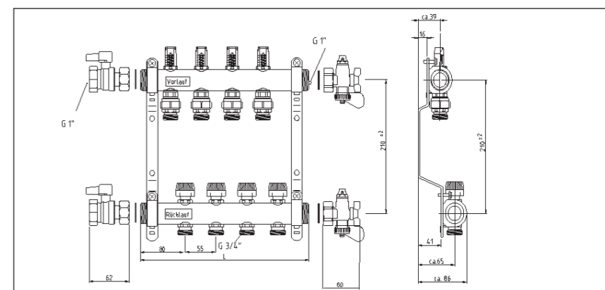
1 Рис. 55: Присоединительные размеры распределительного коллектора НКВ-D
