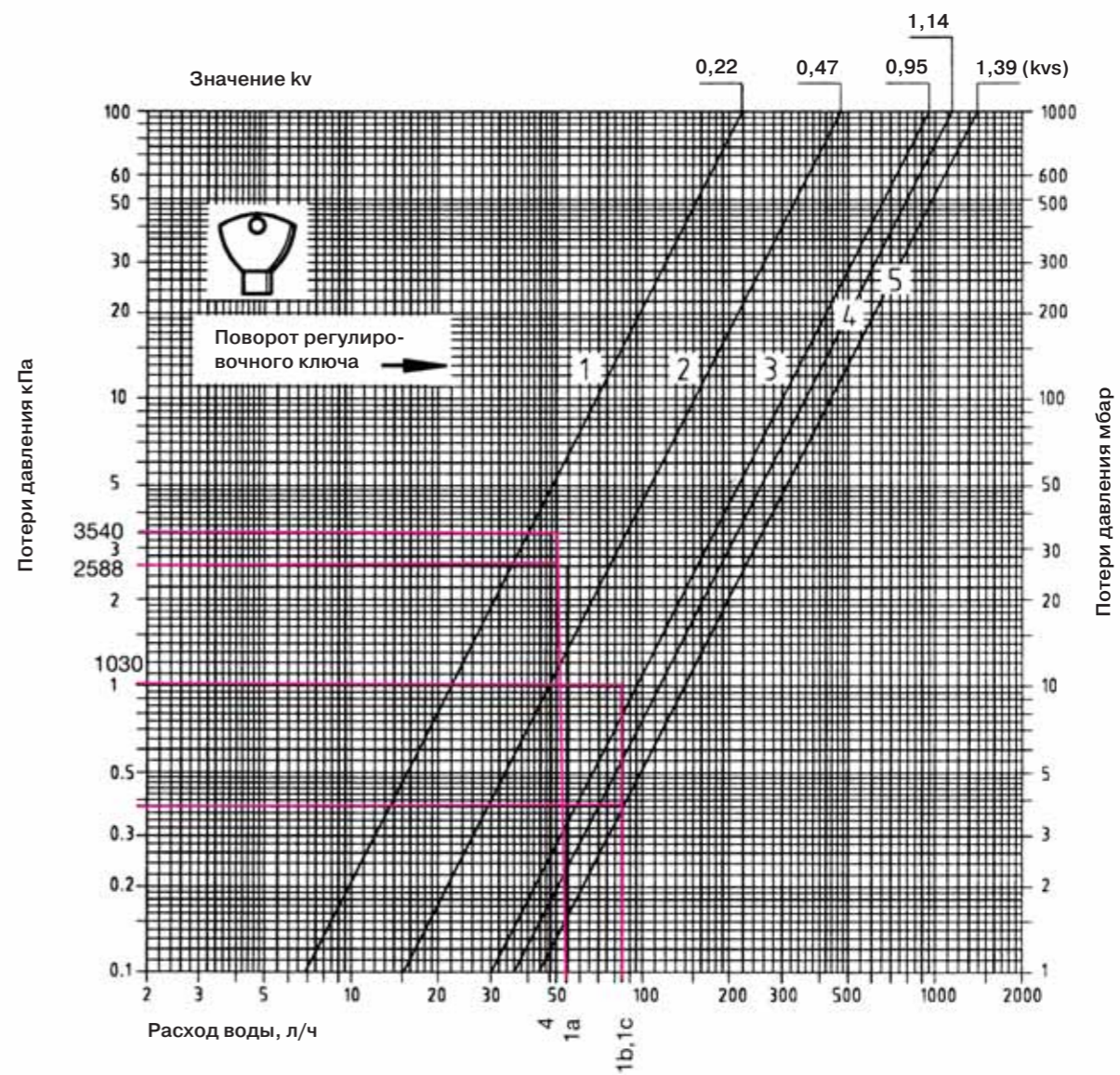
2 Рис. 4: Диаграмма расхода воды для вентиля тонкой регулировки - НКВ
