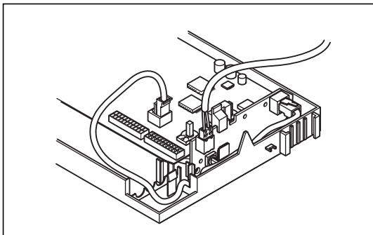
Рис. 4.5 Плата устройства сопряжения с шиной установлена
