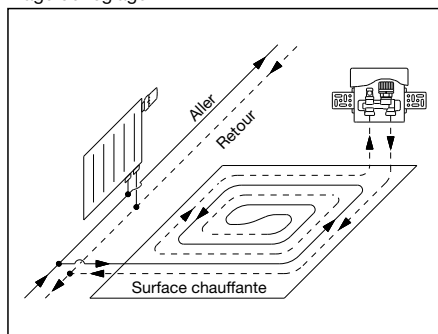
Croquis d'installation
