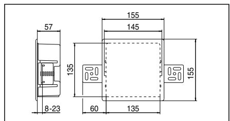
Maße
