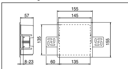
Afmetingen
