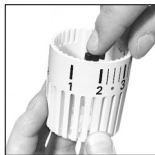
4 Photo 4: Pour limiter la valeur de consigne inférieure, par ex. sur chiffre «2» (environ 16°C), faire glisser un clip dans la nervure devant le chiffre «2» comme sur le photo. (La nervure en face du chiffre «2» reste libre.)
