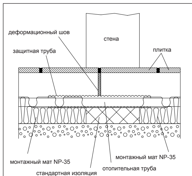
Деформационный шов в дверном проходе
