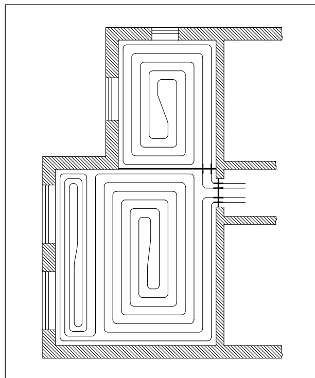
Разделение контуров, устройство деформационных швов
