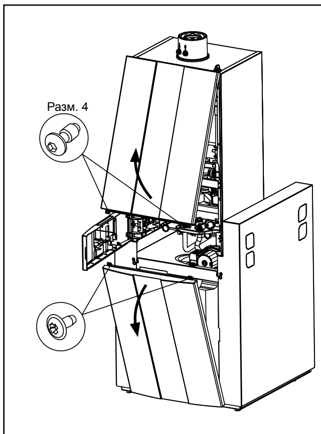
Демонтаж передней обшивки водонагревателя послойного нагрева
