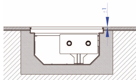
Рис. 21: В правильно установленном конвекторе нащельник находится на уровне напольного покрытия в пределах допуска \pm 1 мм.
