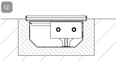
Рис. 20: Очень важно, чтобы вся наружная поверхность конвектора была после этого залита классическим бетоном, вплоть до окончательной высоты черного пола. Теперь конвектор забетонирован в черном полу, который готов к укладке финального покрытия (паркета, плитки и т. д.).
