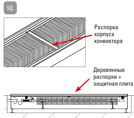
РИС. 18: Чтобы избежать загрязнения ниши во время бетонирования, убедитесь в том, что все отверстия внутри ниши заделаны! Установить в нишу конвектора распорки короба и деревянные распорки вместе с древесноволокнистой защитной плитой конвектора.
