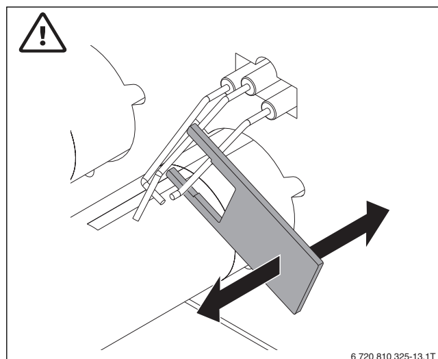
Рис. 66 Проверка расстояния между электродами и стержнем горелки
