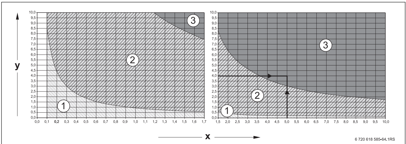
Рис. 54 Допустимое падение давления за одну минуту при контроле внутренней герметичности с имеющимся давлением газа
