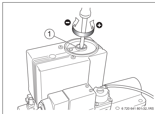
Рис. 37 Корректировка содержания \text{CO}_2 при полной нагрузке на котле мощностью 160 кВт
