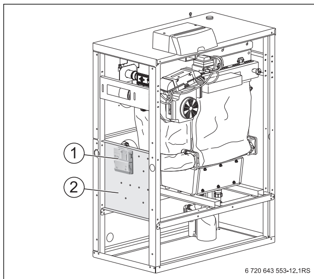
Рис. 21 Установка модулей
