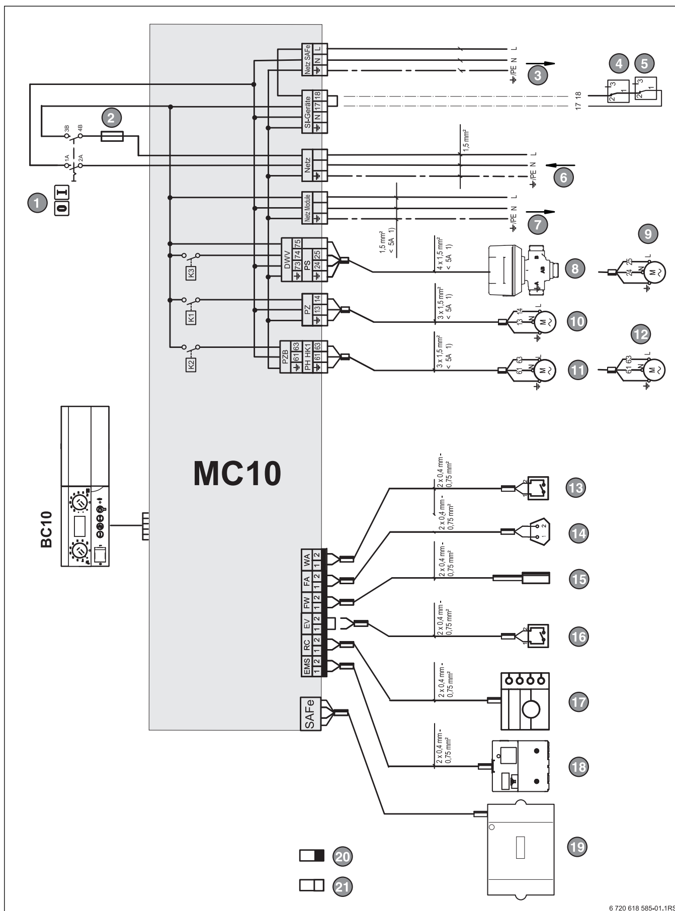
Рис. 75 Схема соединений MC10
