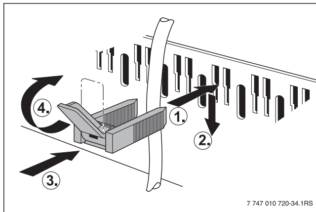
Рис. 23 Крепление электрических проводов хомутами
