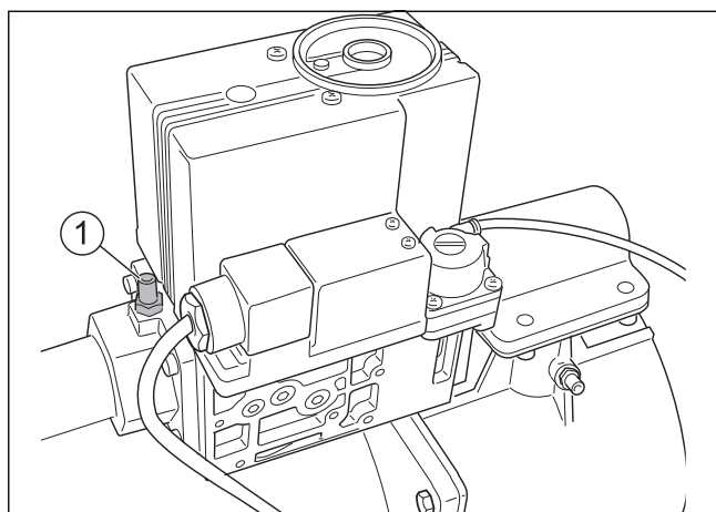
Рис. 45 Измерение подаваемого давления газа на котлах мощностью 160 кВт
