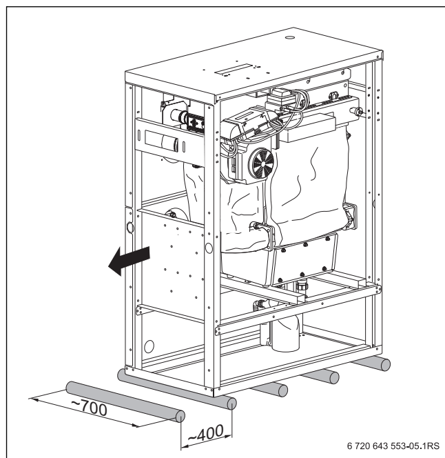
Рис. 6 Перемещение котла перекачиванием на трубах (размеры в мм)
