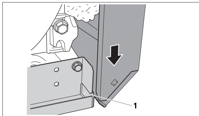
Рис. 41 Установка боковой стенки спереди вниз.
