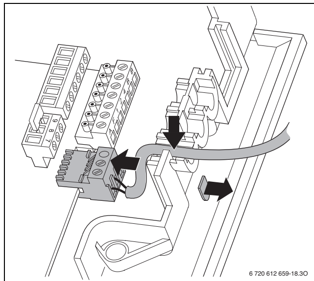
Рис 25 Разъем для подключения датчика температуры емкостного водонагревателя (NTC)
