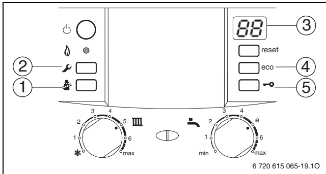
Рис 45 Обзор элементов управления
