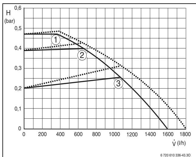
Рис 47 Постоянное давление
