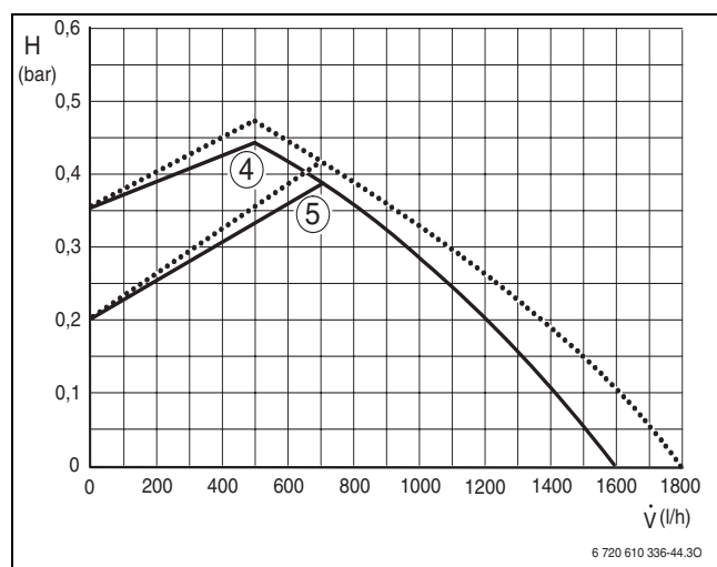
Рис 48 Пропорциональное давление
