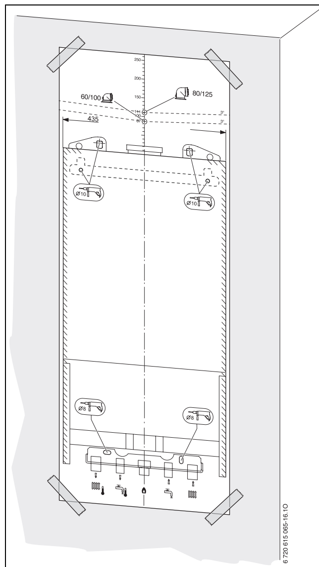
Рис 10 Монтажный шаблон
