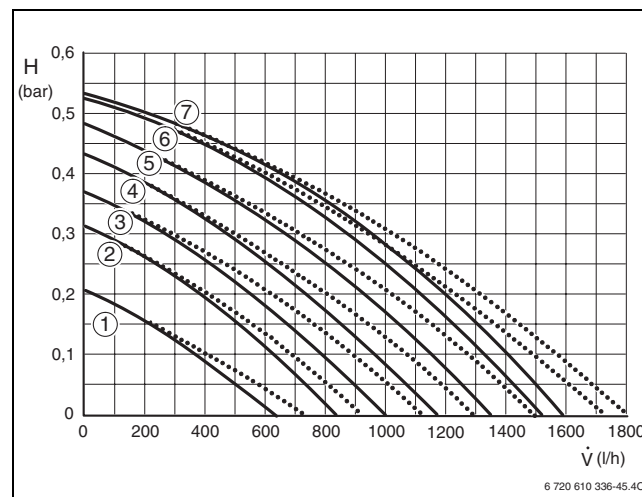
Рис 49 Характеристики насоса в приборах ZSBR
