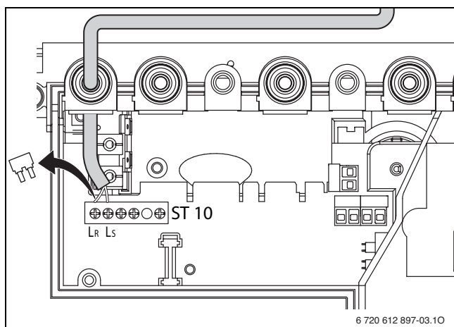
Рис 23 Подключение (230 В AC, снять перемычку между L_S и L_R )
