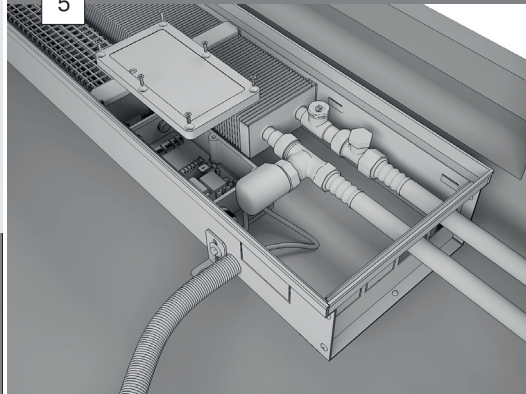
5 ЭЛЕКТРИЧЕСКИЕ ПОДКЛЮЧЕНИЯ
