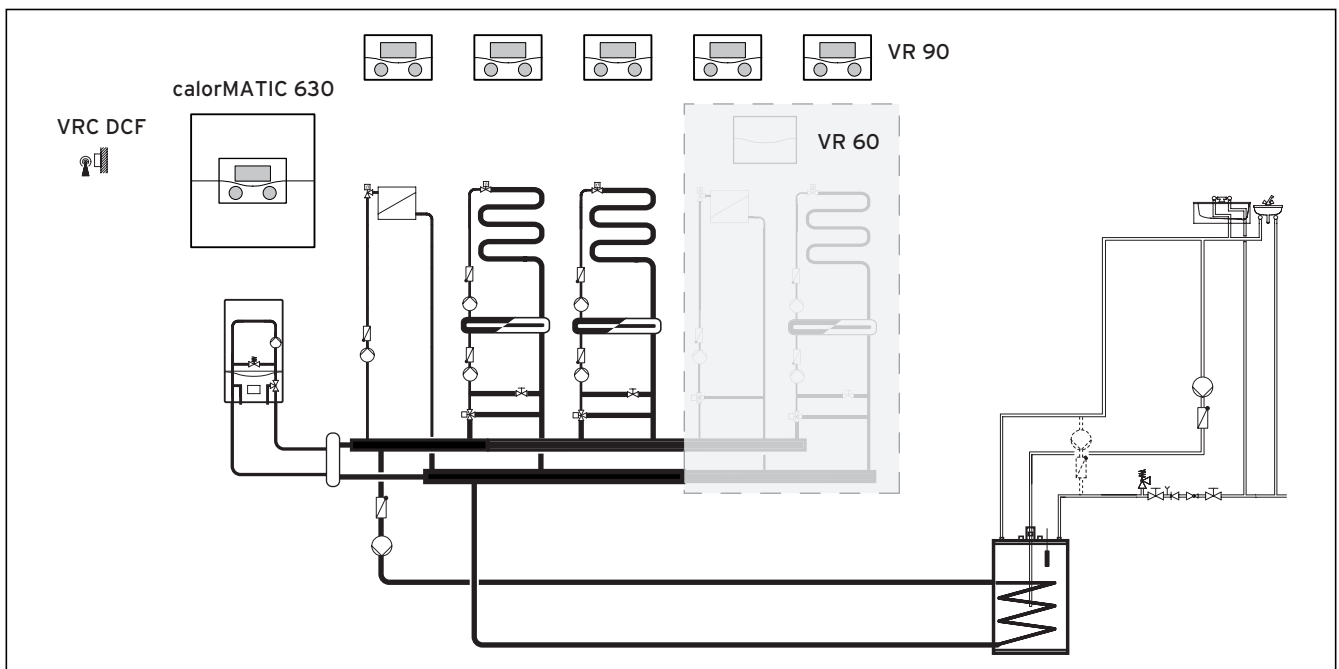
Рис. 3.1 Обзор системы
