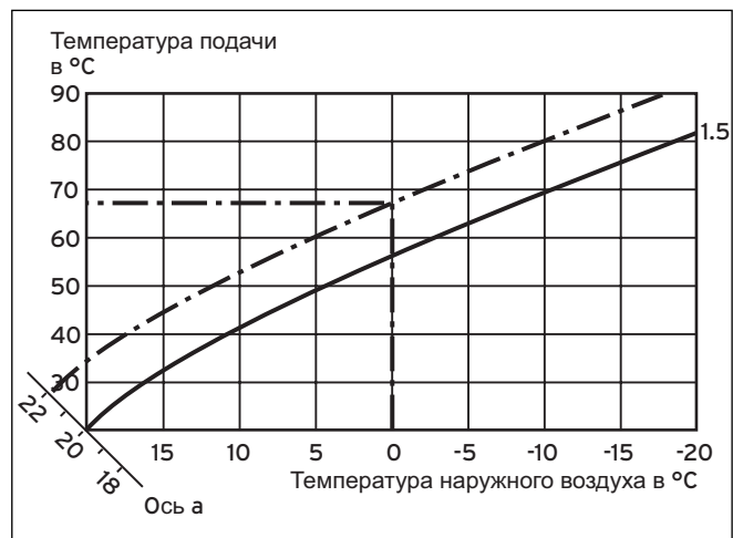
Рис. 3.4 Параллельное смещение отопительной кривой
