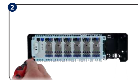
Открутите основную часть корпуса (см. рис.).
