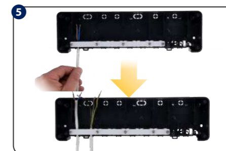
Поведите провода под крепежной планкой в задней части центра коммутации.
