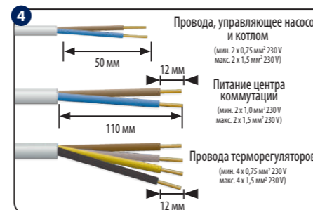
Снимите соответствующие отрезки изоляции проводов.
