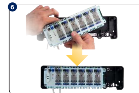
Поведите провода через отверстия в основной части центра коммутации, затем подключите их к клеммам.
