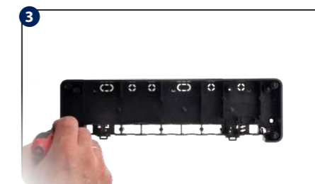
Прикрутите заднюю часть центра коммутации к стене (если монтируете центр коммутации на DIN-рейке - зафиксируйте его с помощью крепежа находящегося на задней части корпуса).
