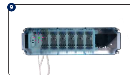
Убедитесь, что все провода подключены правильно, затем прикрутите верхнюю крышку и подключите питание 230 V - зелёный светодиод "Power" засветится.
