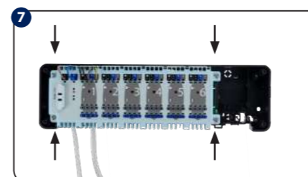
Убедитесь, что все провода подключены правильно, затем прикрутите основную часть корпуса.
