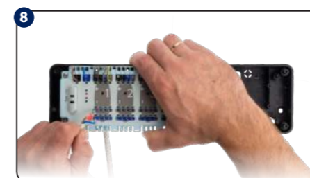
Подключите провода сервоприводов.
